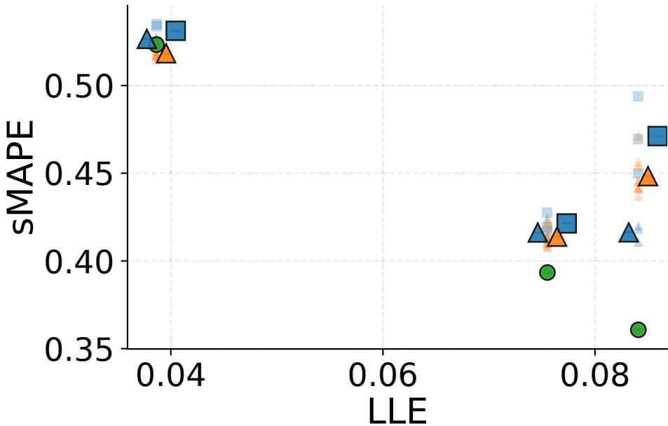
sMAPE: PEMS
