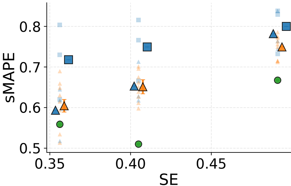
sMAPE: Fitbit
