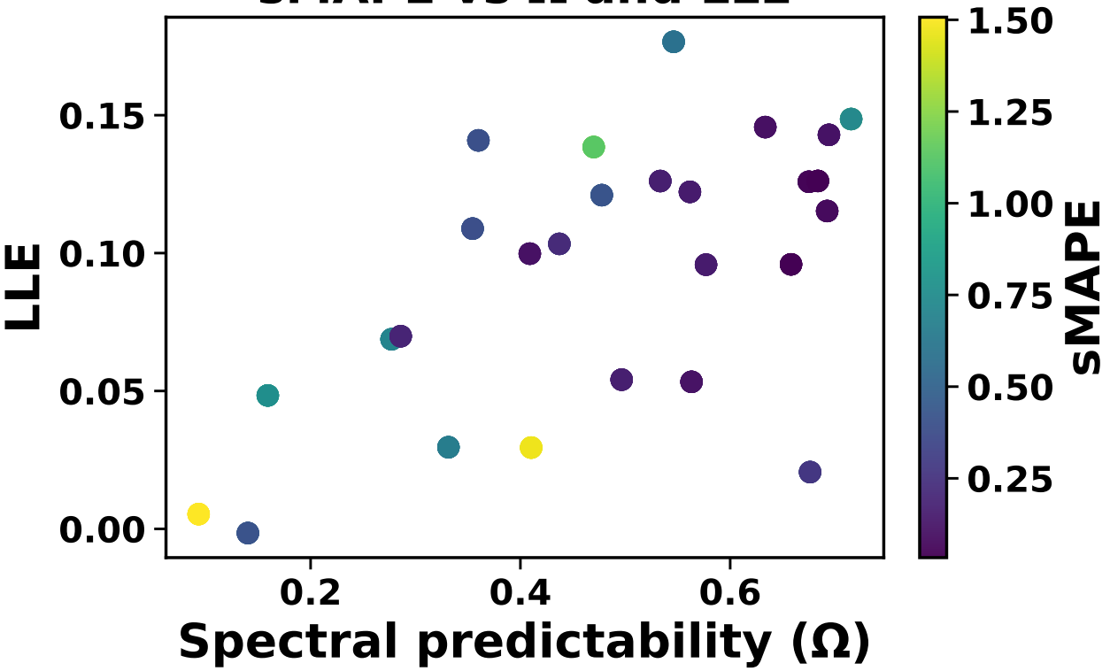
sMAPE vs \Omega and LLE
