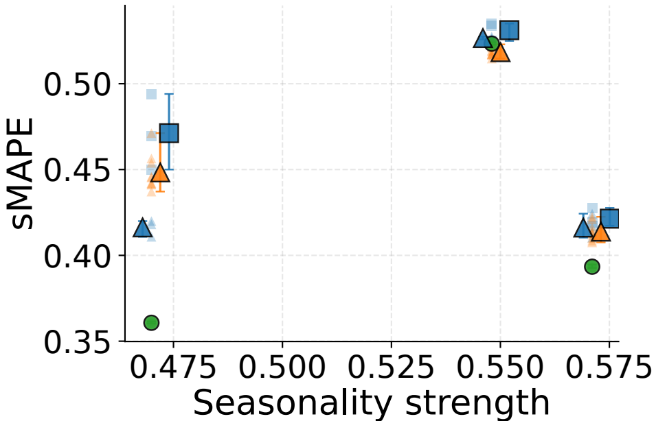
sMAPE: PEMS
