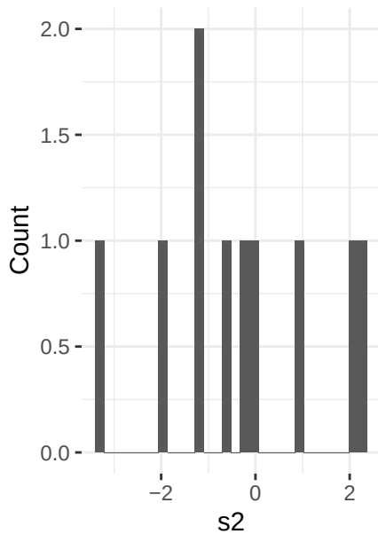
s2 Posterior
