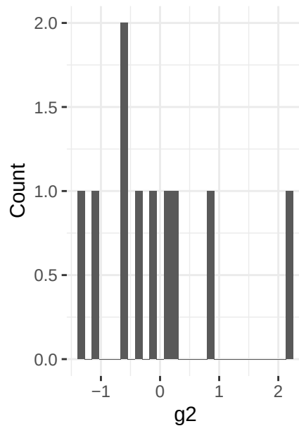
g2 Posterior
