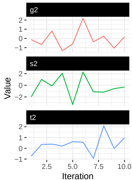
g2 Posterior
