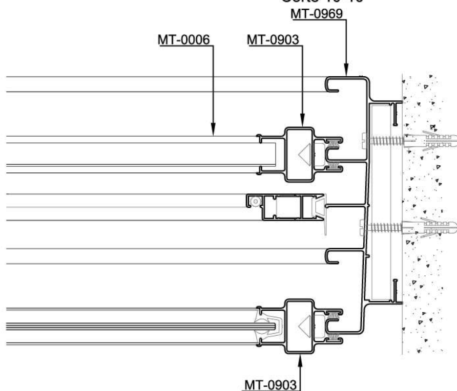
Corte 10-10
