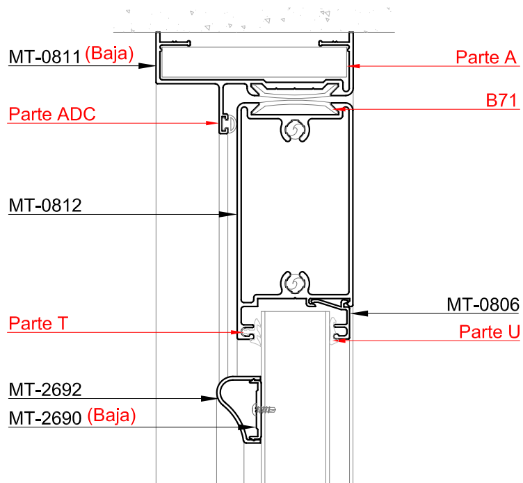
Corte 1-1
