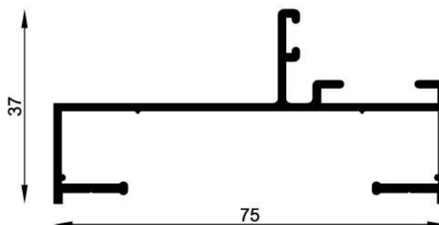
MT-0950 Marco recto Peso estimado: 0.651 Kg/m Largo STD: 6150 mm
