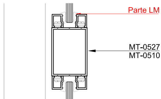
Corte 8"-8"
