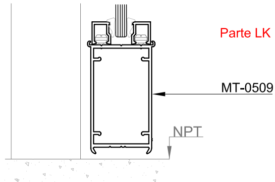
Corte 9"-9"
