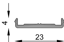
MT-2690 Base moldura puerta placa Peso estimado: 0.116 Kg/m Largo STD: 6030 mm Baja, consultar stock con distribuidor.
