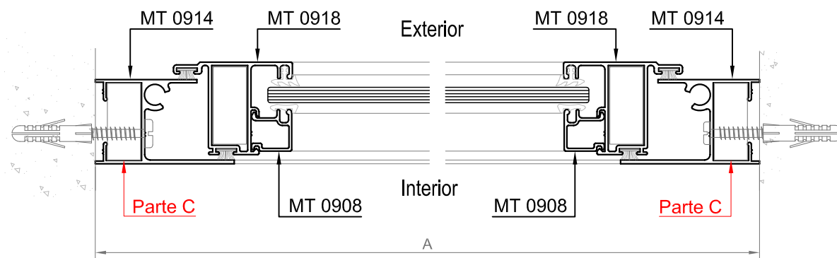
Corte 3-3
