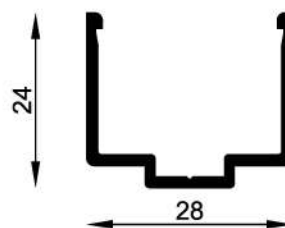
MT-0919 Adaptador para DVH h. corredizas Peso estimado: 0.273 Kg/m Largo STD: 6030 mm
