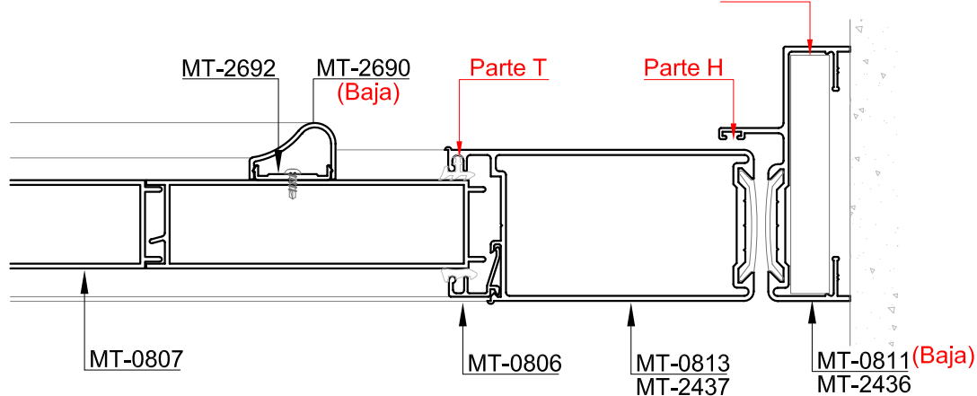
Corte 5-5 Parte A
