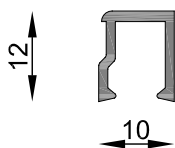
MT-0507 Contravidrio Peso estimado: 0.111 Kg/m Largo STD: 6030 mm Baja, consultar stock con distribuidor.
