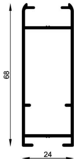
MT-0951 Parante Hoja Peso estimado: 0.645 Kg/m Largo STD: 6150 mm
