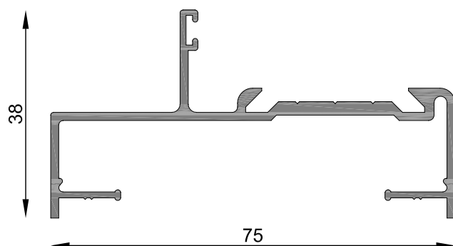
MT-0811 Marco de puerta encolizada Peso estimado: 0.761 Kg/m Largo STD: 6150 mm Baja, consultar stock con distribuidor.
