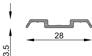
MT-0511 Tapacanto puerta de rebatir Peso estimado: 0.103 Kg/m Largo STD: 6030 mm Baja, consultar stock con distribuidor.
