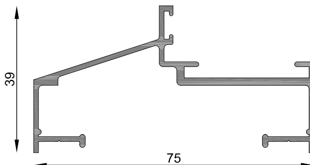
MT-2740 Marco puerta 36mm y celosia regulable Peso estimado: 0.740 Kg/m Largo STD: 6150 mm
