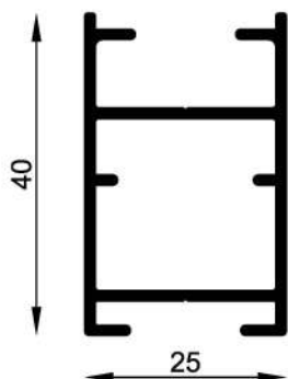
MT-2733 Batiente puerta rebatir Peso estimado: 0.483 Kg/m Largo STD: 6150 mm
