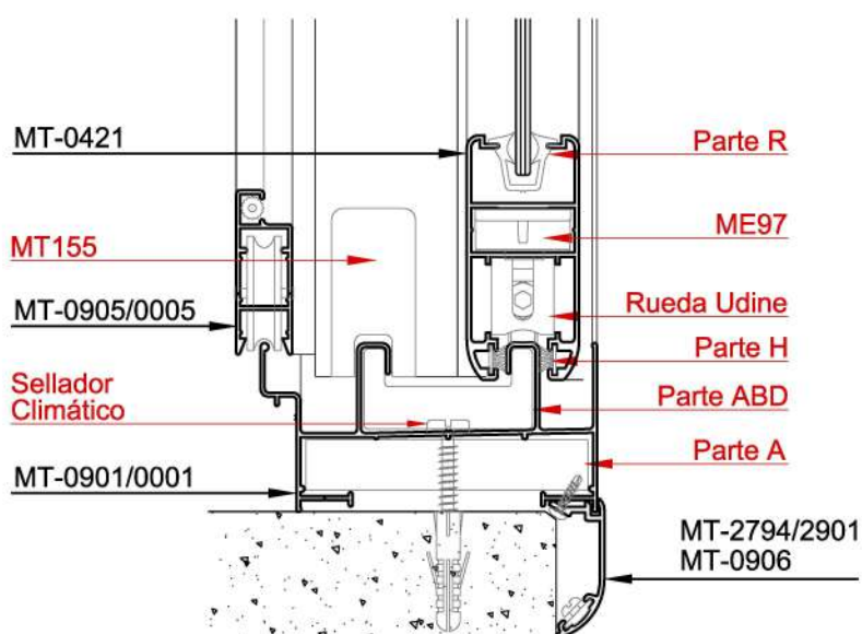
Corte 2-2
