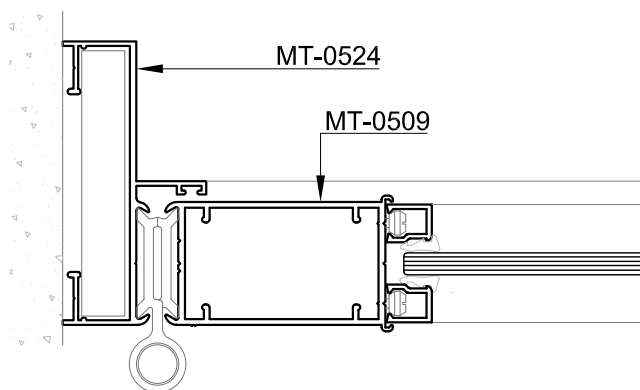
Corte 10"-10"
