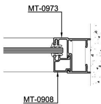
Corte 11-11
