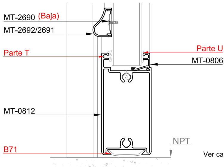
Corte 3-3
