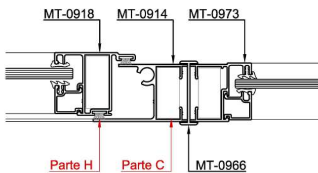
Corte 10-10
