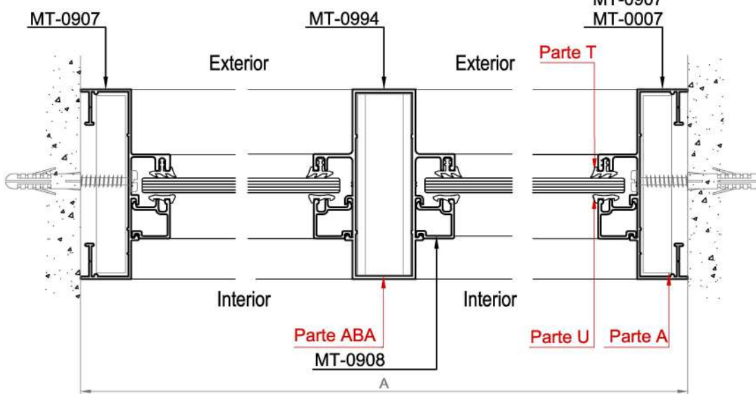
Corte 4-4
