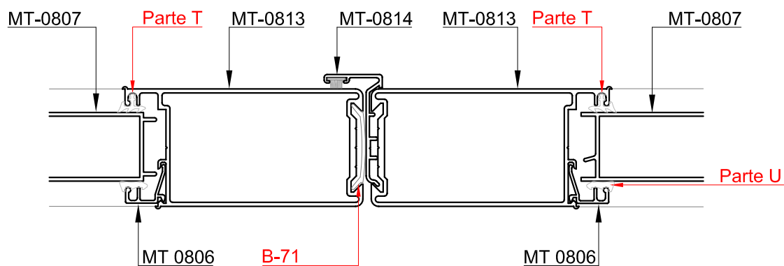
Corte 6-6
