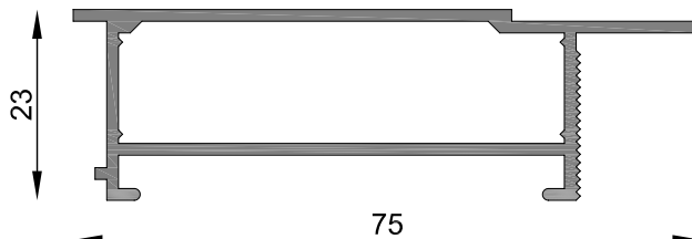
MT-0954 Premarco Peso estimado: 0.697 Kg/m Largo STD: 6150 mm Baja, consultar stock con distribuidor.
