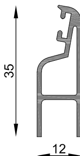
MT-2706 Terminal corto celosía regulable Peso estimado: 0.305 Kg/m Largo STD: 6030 mm
