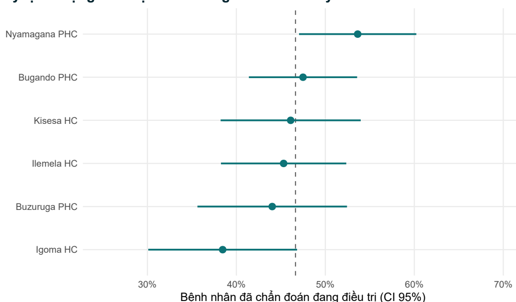
Hình 3.3: Tỷ lệ bệnh nhân tăng huyết áp đã được chẩn đoán đang điều trị tại mỗi cơ sở y tế, kèm khoảng tin cậy 95%; đường nét đứt đánh dấu tỷ lệ chung (46,6%). Các cơ sở được sắp xếp theo tỷ lệ sử dụng điều trị.
