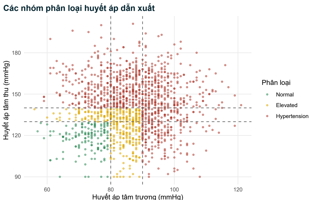
Hình 2.4: Huyết áp tâm thu theo huyết áp tâm trương, tô màu theo phân loại huyết áp dẫn xuất. Các đường nét đứt đánh dấu ngưỡng 130/80 và 140/90 mmHg; các nhóm tạo thành những vùng hình chữ L như mong đợi.
