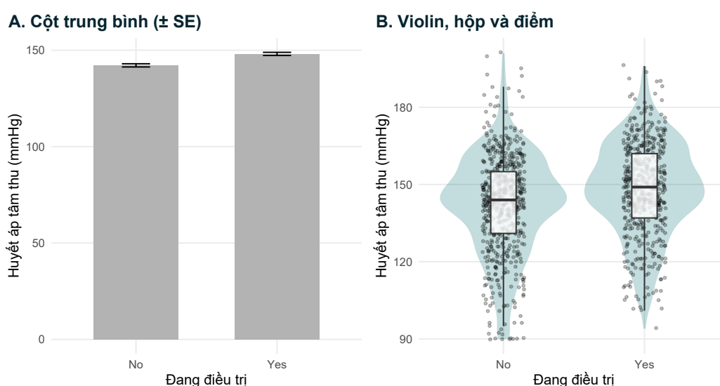
Hình 3.6: Cùng một dữ liệu SBP của bệnh nhân đã được chẩn đoán được trình bày theo hai cách: (A) biểu đồ cột của trung bình kèm thanh sai số chuẩn che giấu phân phối; (B) biểu đồ violin kèm biểu đồ hộp và từng bệnh nhân (các điểm được rải ngẫu nhiên) cho thấy toàn bộ độ phân tán, sự chồng lấp giữa các nhóm và mọi giá trị ngoại lai.
