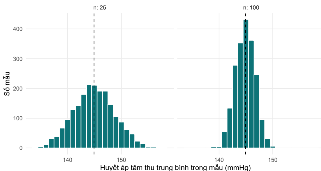
Hình 4.1: Phân phối mẫu của huyết áp tâm thu trung bình trong 2.000 mẫu ngẫu nhiên gồm 25 và gồm 100 bệnh nhân đã được chẩn đoán. Mẫu lớn hơn cho các trung bình tập trung sát hơn quanh trung bình quần thể (đường nét đứt).
