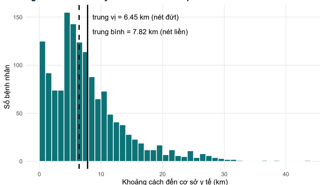
Khoảng cách đến cơ sở y tế có đuôi dài bên phải
