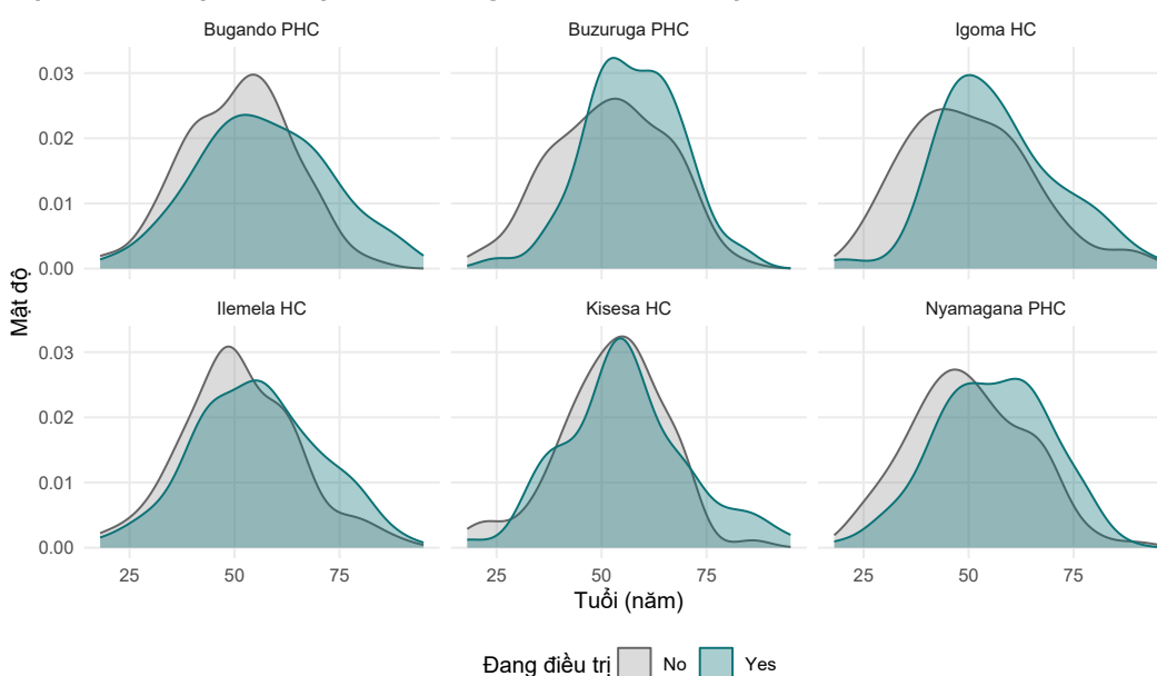
Bệnh nhân được điều trị có xu hướng lớn tuổi hơn ở mọi cơ sở
