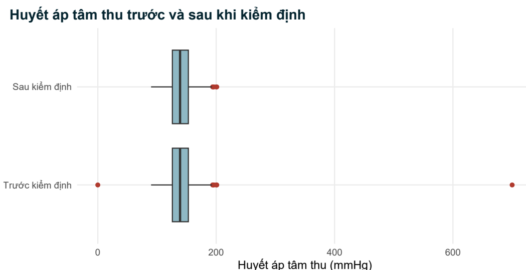
Hình 2.2: Huyết áp tâm thu trước và sau khi kiểm định. Trước khi kiểm định, các giá trị 0 và 700 mmHg kéo giãn trực vượt xa phạm vi của dữ liệu hợp lý; sau khi kiểm định, phân phối hợp lý về mặt lâm sàng.
