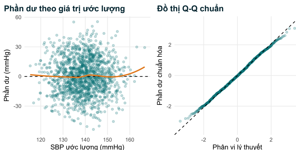
Hình 5.1: Chẩn đoán phần dư cho mô hình hồi quy tuyến tính của huyết áp tâm thu theo tuổi và BMI. Trái: phần dư theo giá trị ước lượng, kèm đường cong làm trơn; phải: đồ thị Q-Q chuẩn của phần dư.
