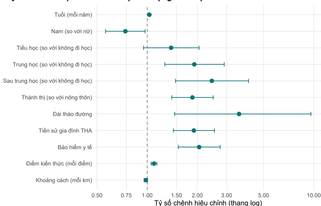
Hình 5.5: Biểu đồ rừng của các tỷ số chênh hiệu chỉnh (khoảng tin cậy 95%) cho việc sử dụng điều trị từ mô hình hồi quy logistic đa biến ( n = 992 ). Trục hoành dùng thang logarit; đường nét đứt đánh dấu OR = 1 .
