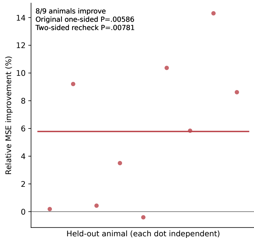
B · VTA Post DA: belief surprise
