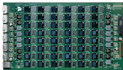
SpiNNaker 2
