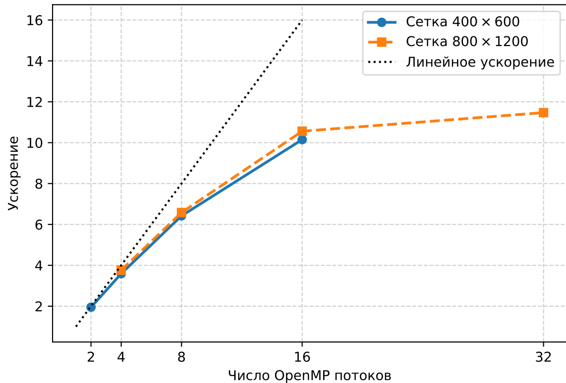
Ускорение
