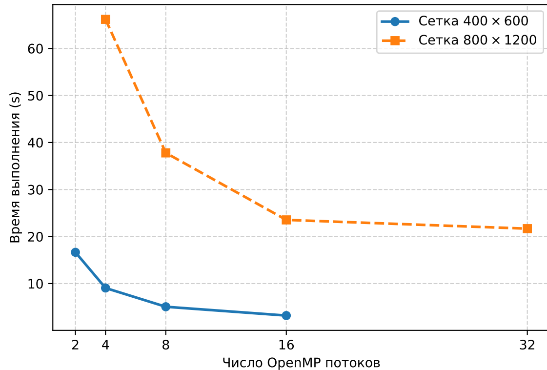
Время выполнения
