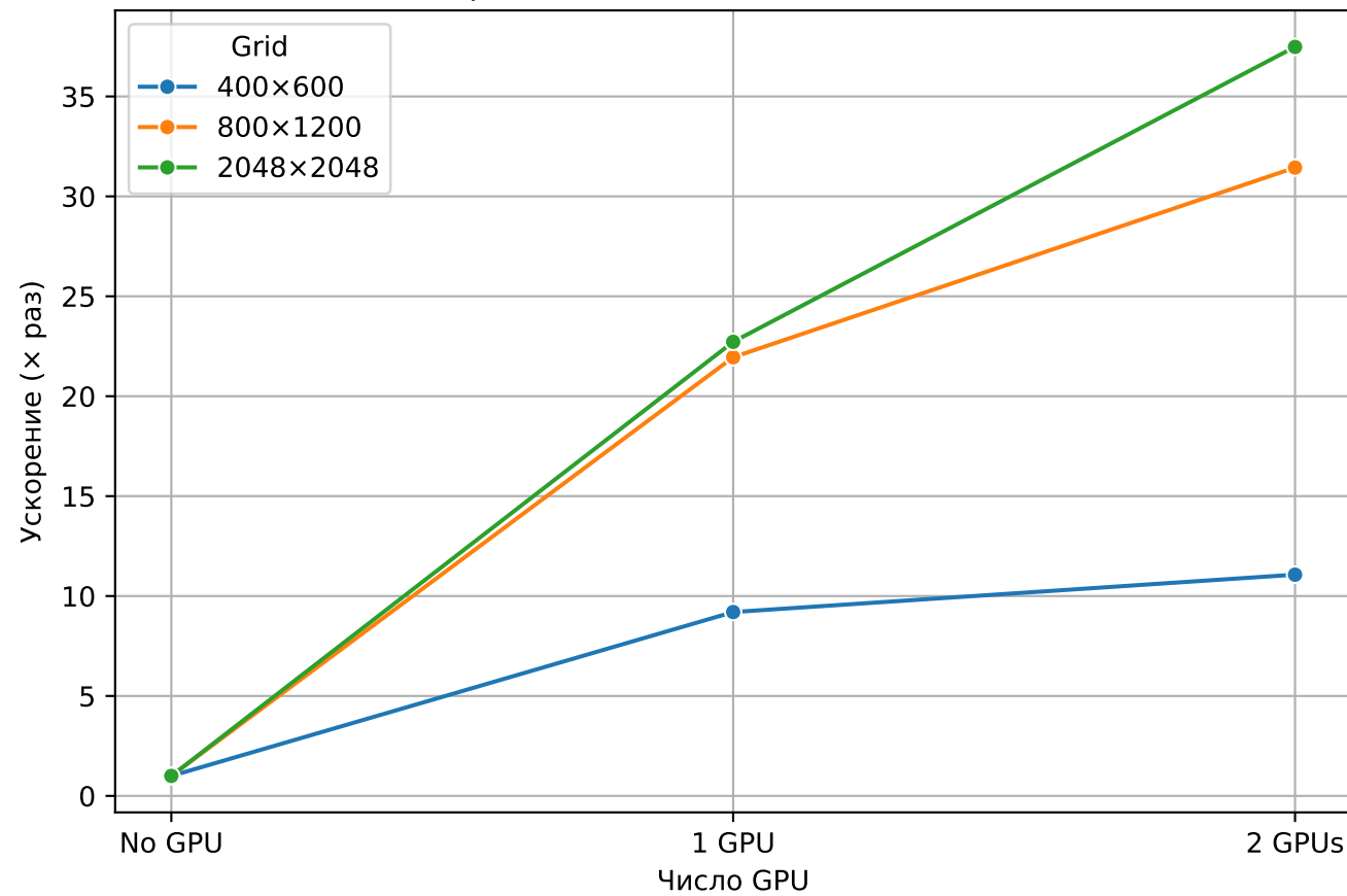
Ускорение в зависимости от числа GPU
