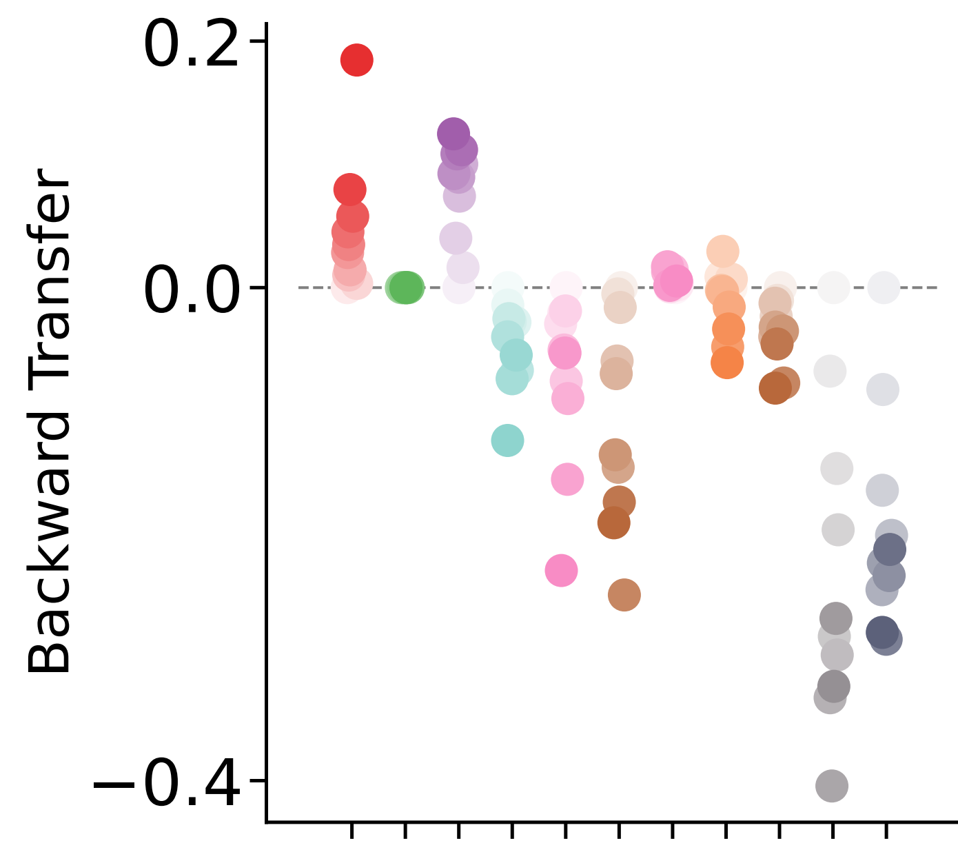
CIFAR 10X10 (500 samples per task)
