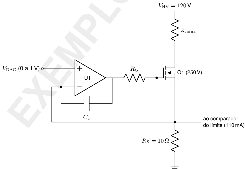
Figura 2 – A fonte de corrente de um canal. A tensão em R_S também alimenta o comparador do limite de corrente. Fonte: Elaborado pela autora.
