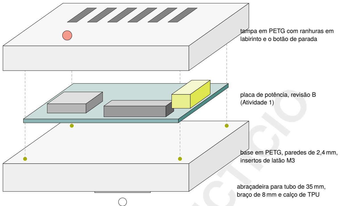
Figura 7 – Vista explodida do invólucro: a base com a abraçadeira, a placa e a tampa. Fonte: Elaborado pela autora.
