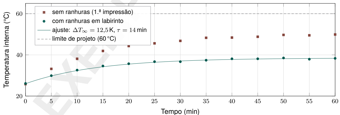
Figura 8 – Temperatura do ar dentro do invólucro em estimulação contínua na amplitude máxima, a 26 °C de ambiente. Fonte: Relatório de execução NRO-PRO-003-902.
