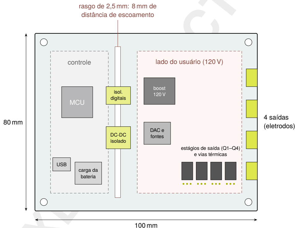
Figura 3 – Planta simplificada do layout da revisão B: as áreas, a barreira de isolamento e os estágios de saída. O layout completo está no repositório.
