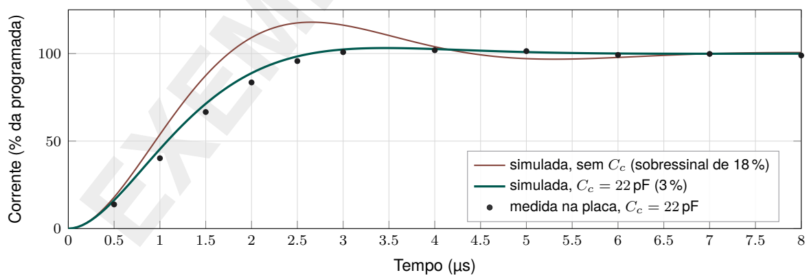
Figura 6 – A borda de subida da corrente: simulada sem e com a compensação, e medida na placa. Fonte: Elaborado pela autora.
