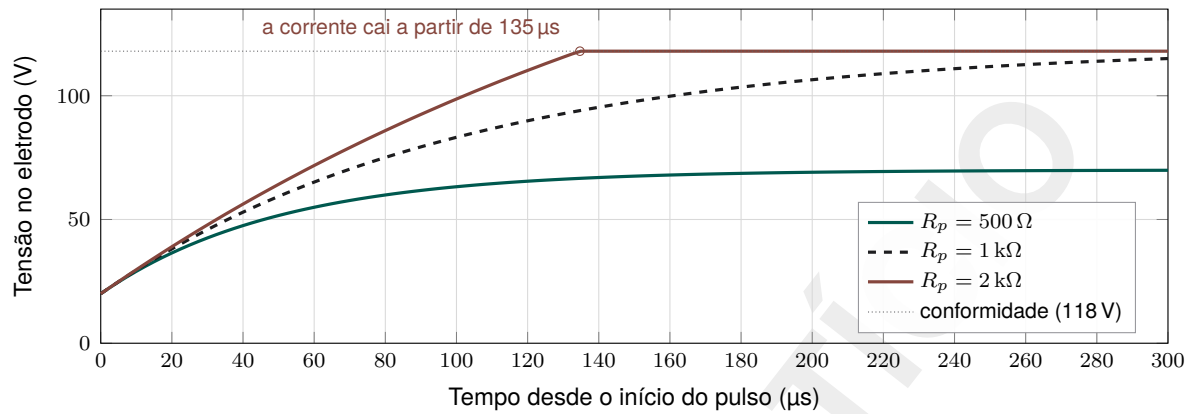
Figura 5 – Tensão no eletrodo durante um pulso de 100 mA, para três valores de R_p , com a alimentação de 120 V. Fonte: Elaborado pela autora (simulação, eq. 3).
