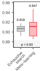
AUPRC
