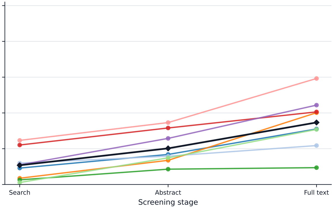
Precision
