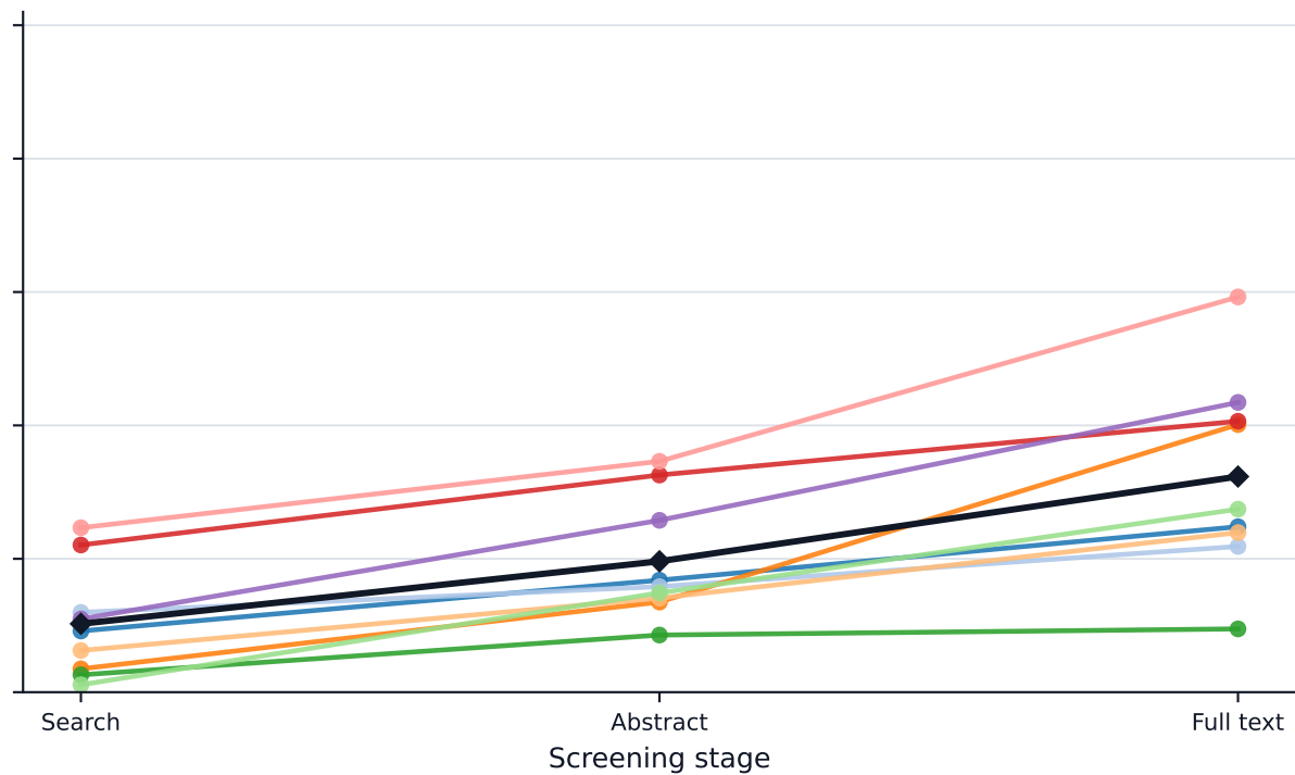
Precision
