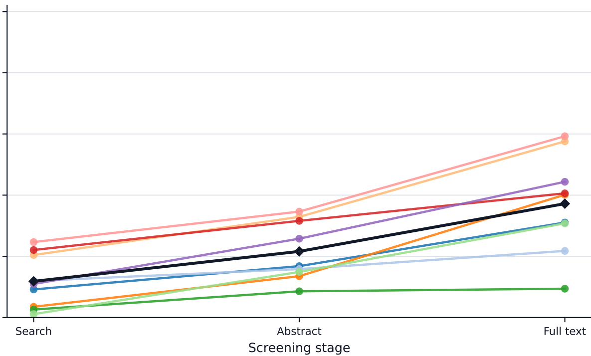
Precision
