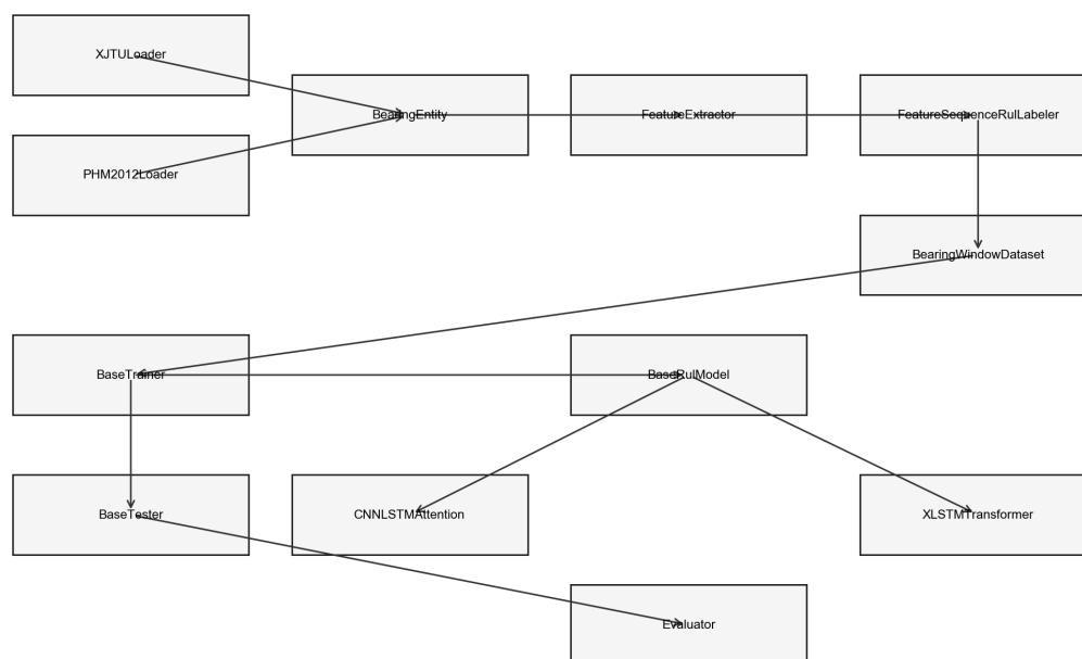
Figure 2: UML 核心类图
