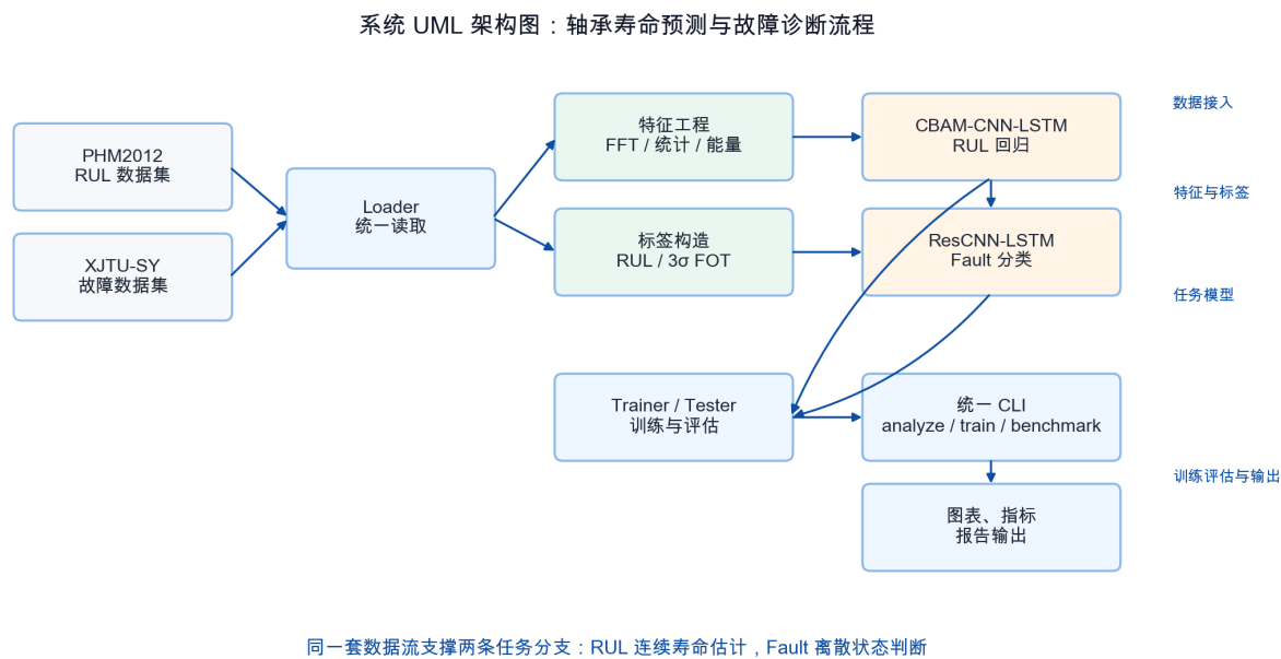
Figure 1: 系统 UML 架构图
