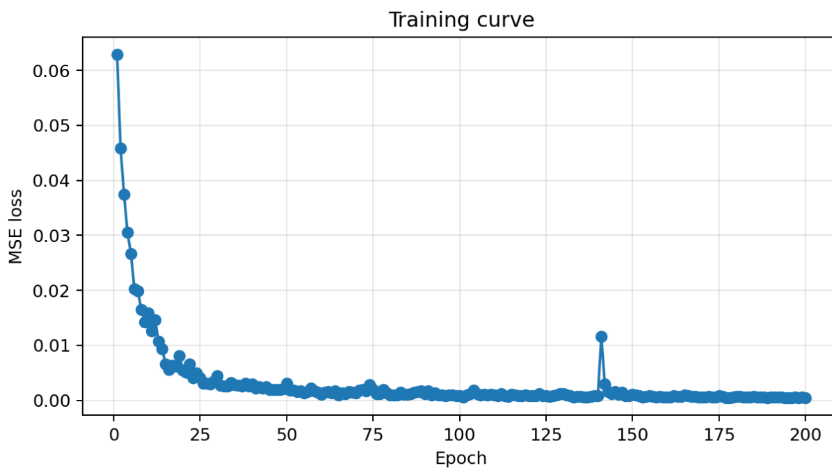
Figure 4: 训练/验证指标图
