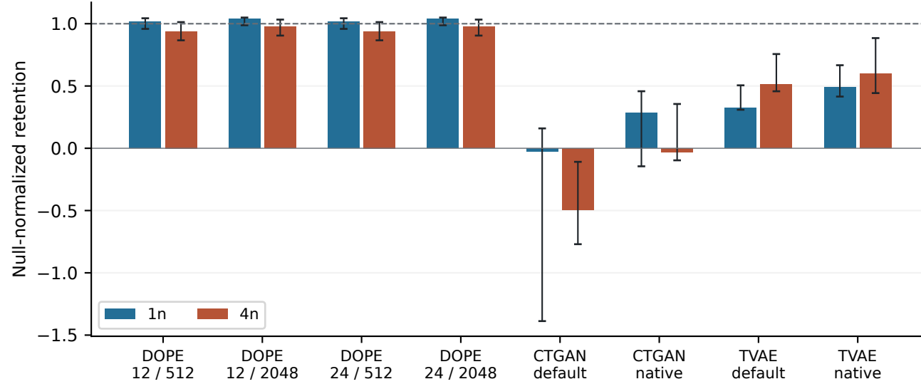
210_cloud 0d482c1dd7cc6592
