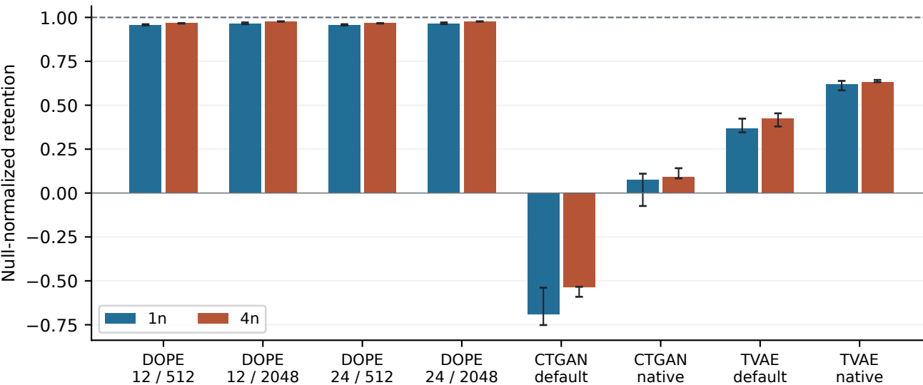
feynman_test_11 471f11cc2d38853a
