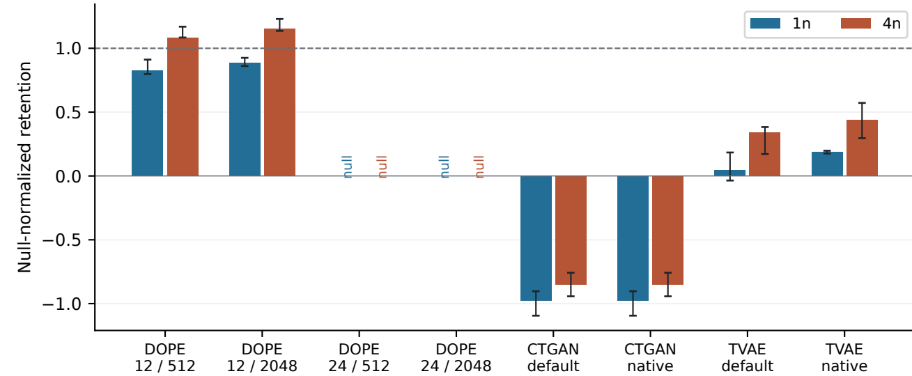
603_fri_c0_250_50 297b7688a045c583
