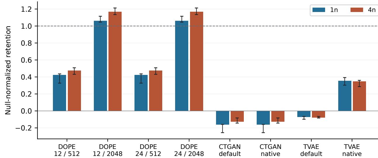
feynman_test_1 1a4456d1cc71a26a
