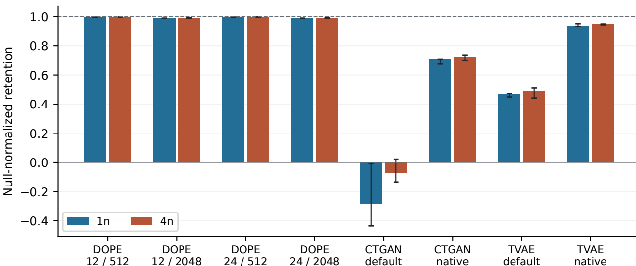
feynman_l_12_1 642738a361f1c63a
