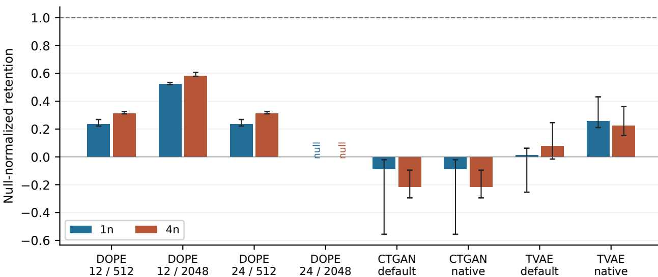
strogatz_vdp1 ed2efb82fce4b098
