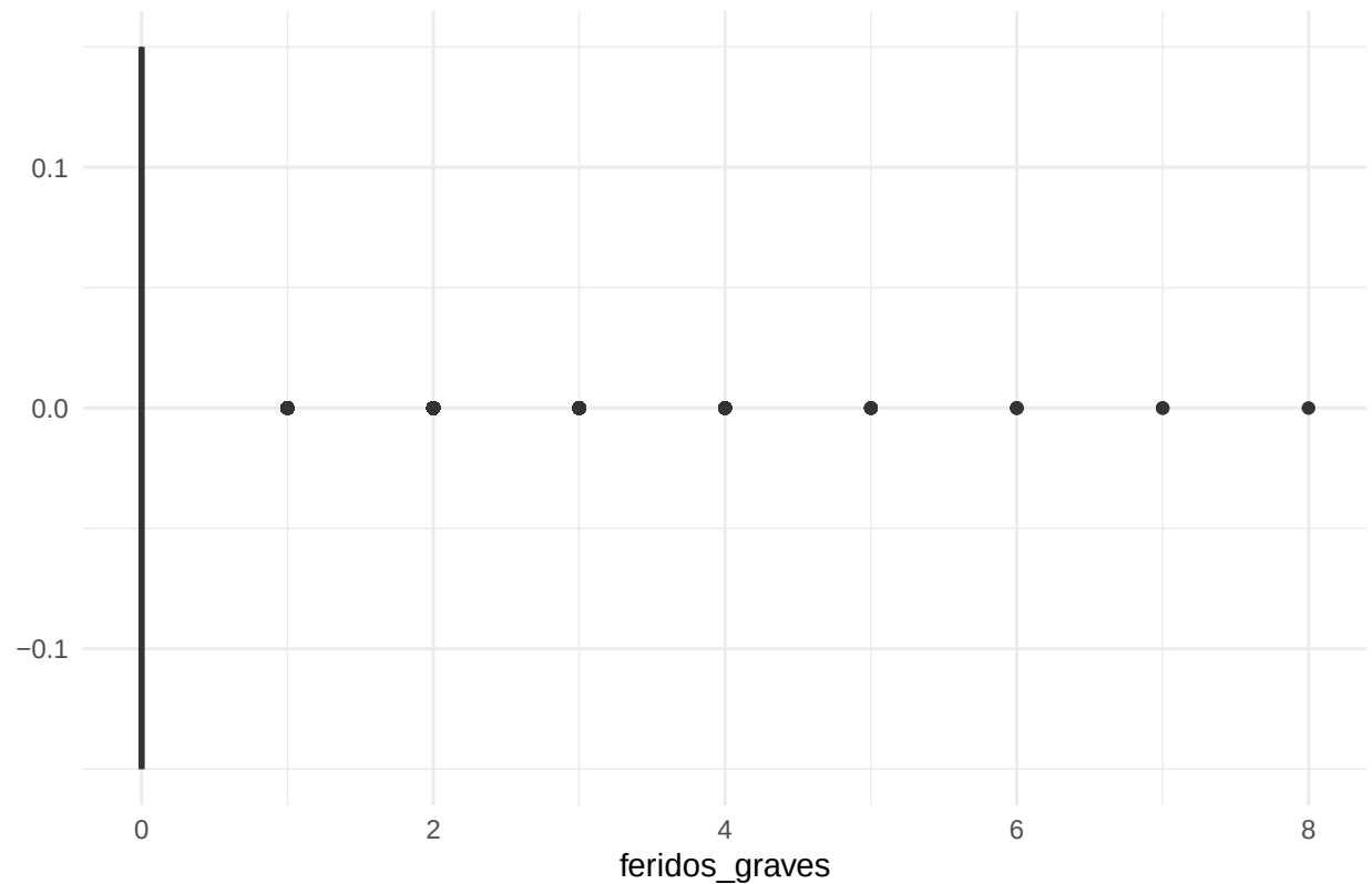
Boxplot de feridos_graves
