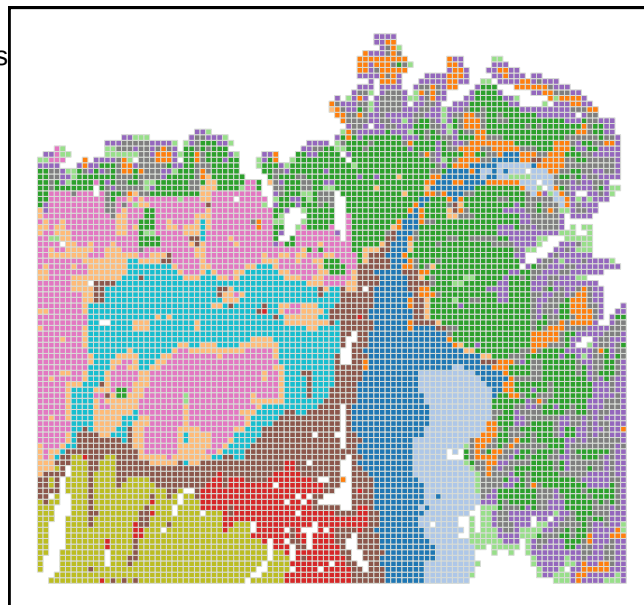
DRSC
