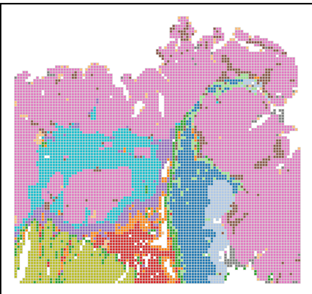
BNPMFA
