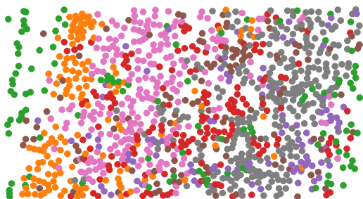
SpaGCN: ARI=0.229
