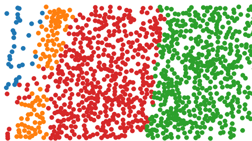
DRSC: ARI=0.347
