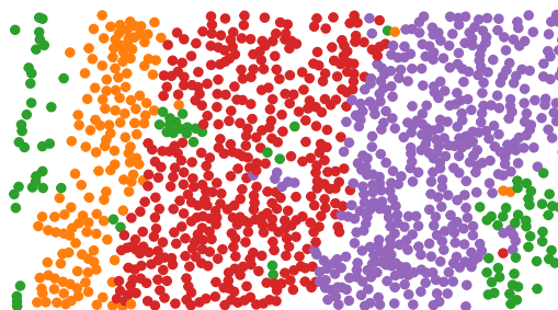
ADEPT: ARI=0.664
