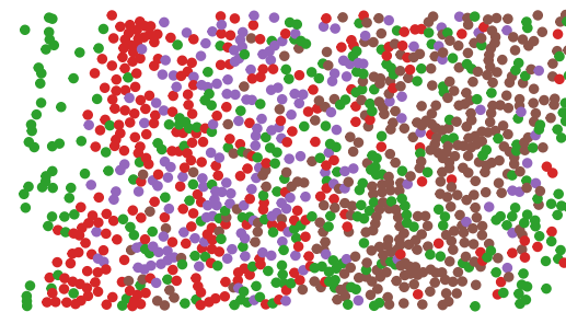
Louvain: ARI=0.181
