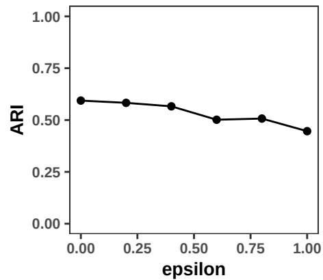
151669
