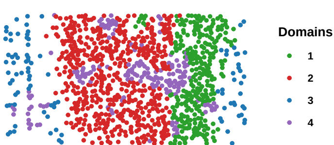
ADEPT: ARI=0.459
