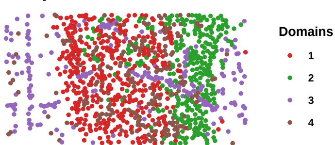
SpaGCN: ARI=0.256
