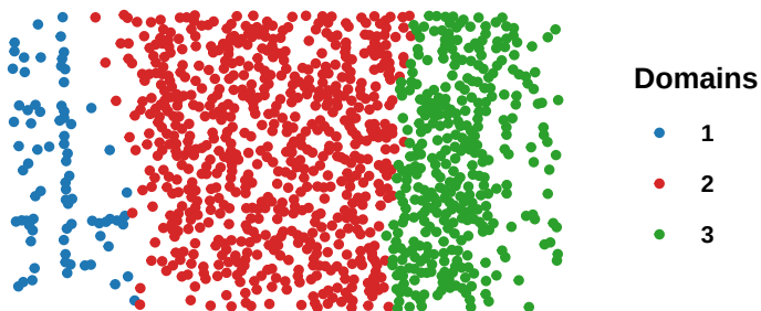
DRSC: ARI=0.309
