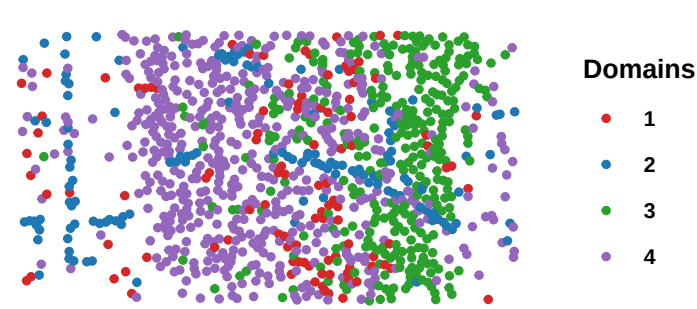
Louvain: ARI=0.195
