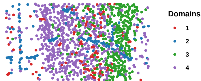
Louvain: ARI=0.195
