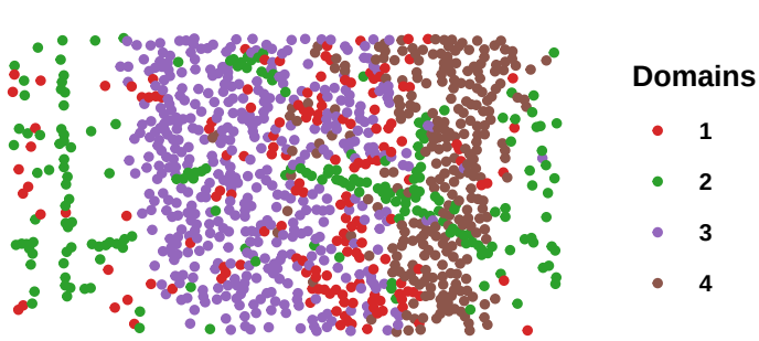
DRSC: ARI=0.309
