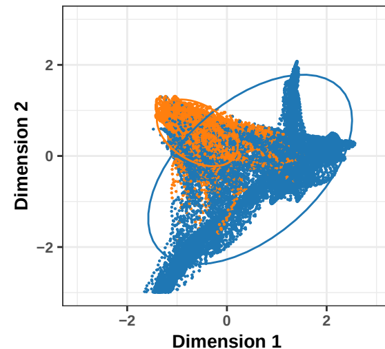
SpatialPCA Embedding
