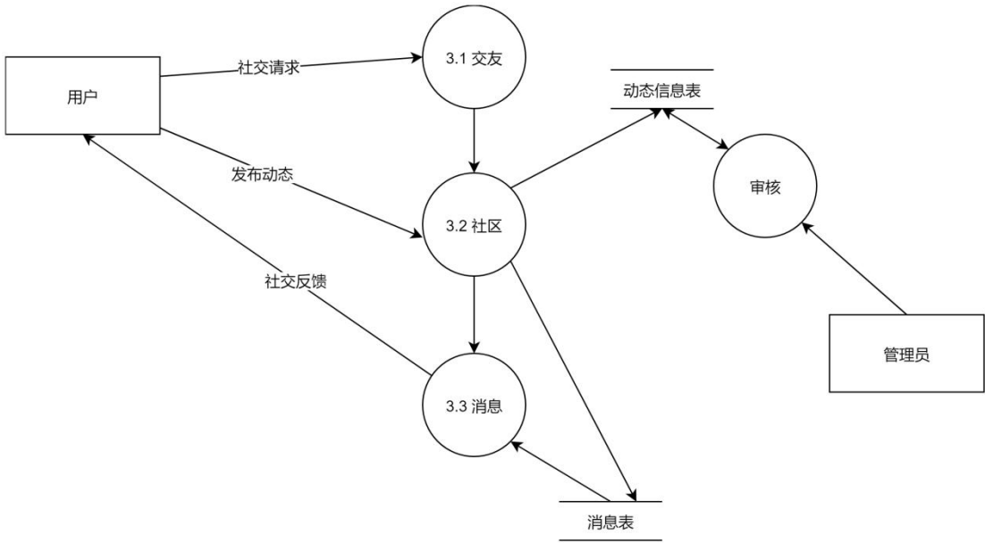
图 B-4 社交功能数据流图
