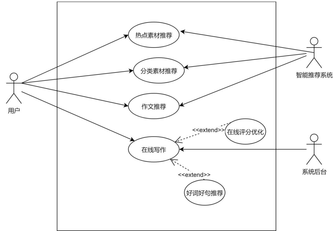
图 4-2 作文相关功能用例图
