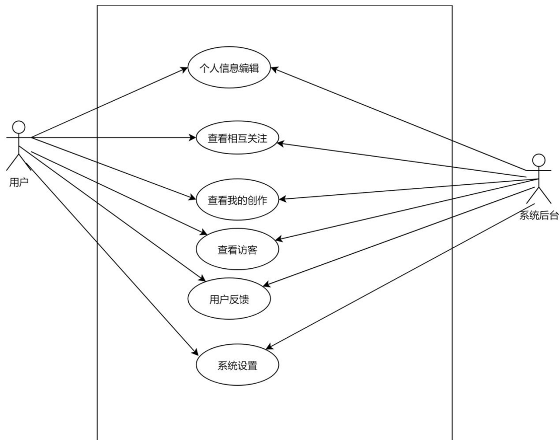
图 4-5 我的界面功能用例图
