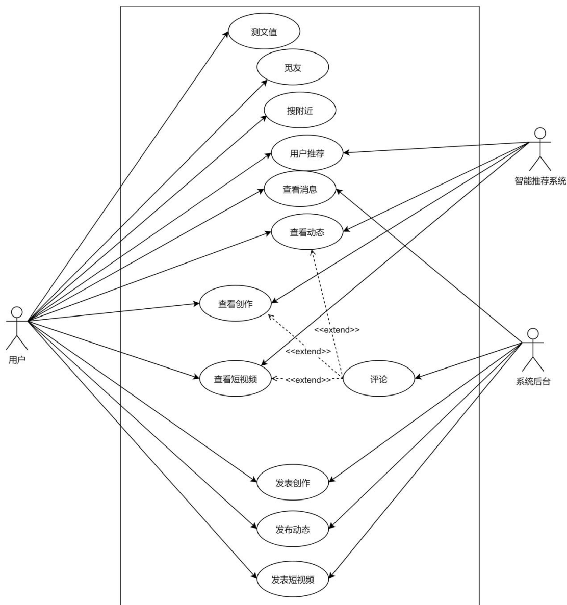
图 4-3 社交功能用例图
