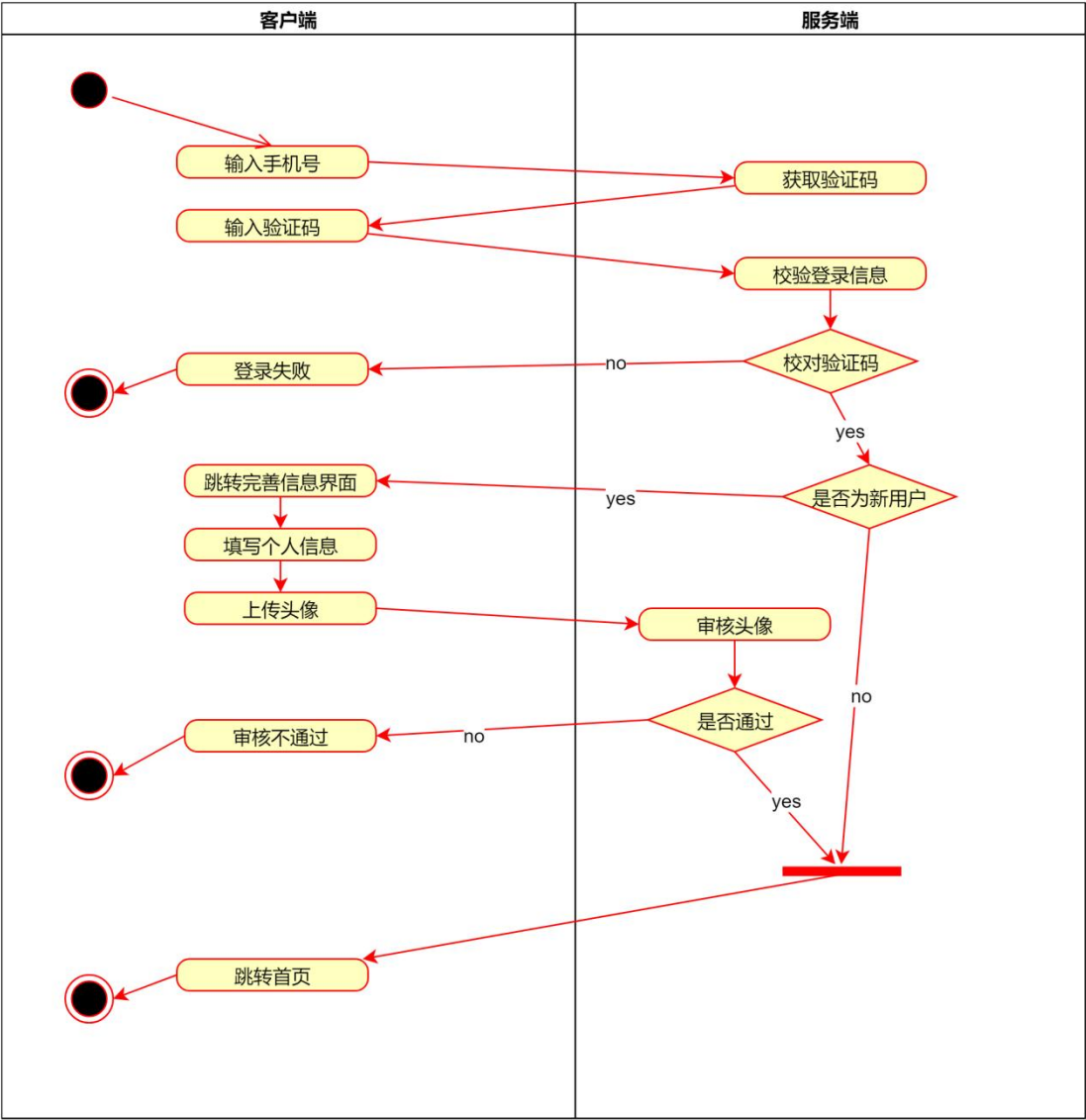
图 B-11 单点登陆活动图
