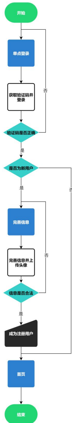
图 B-6 单点登陆业务流程图
