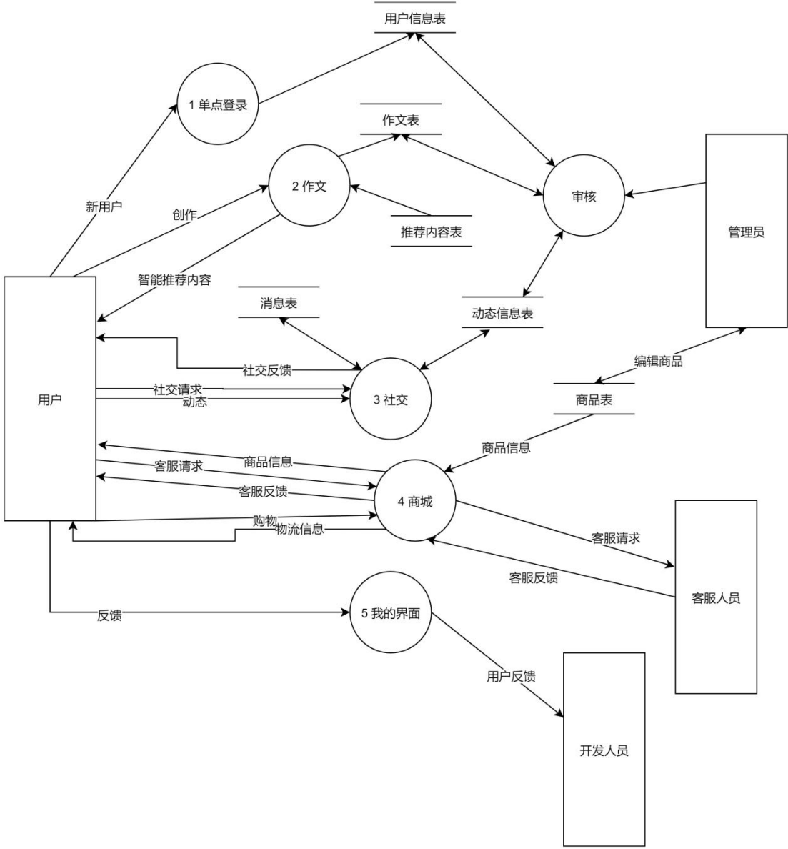
图 B-2 1-层数据流图
