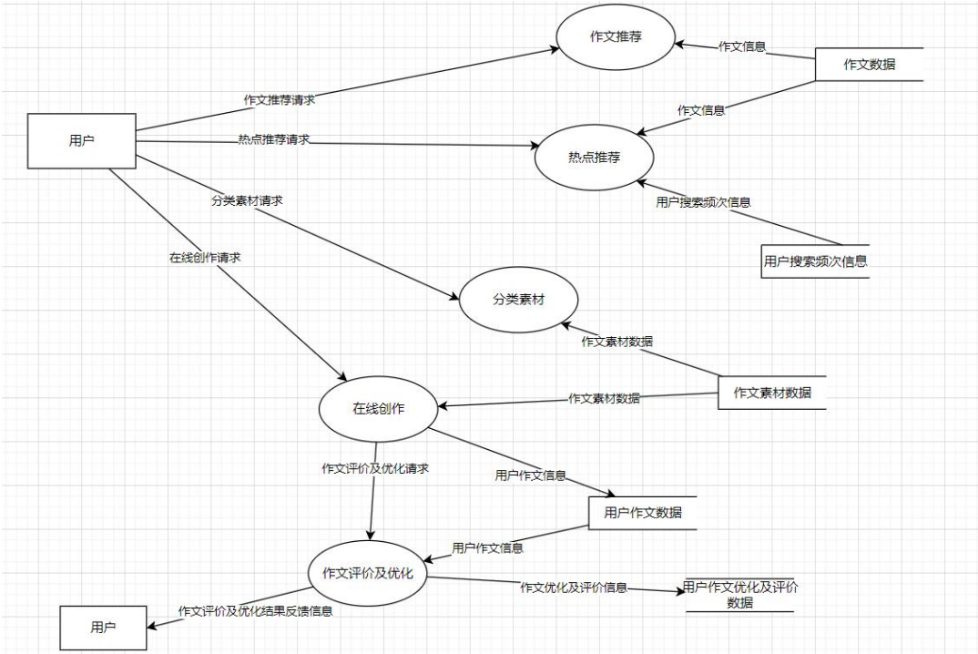
图 B-3 作文功能数据流图
