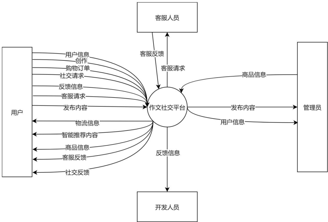
图 B-1 0-层数据流图
