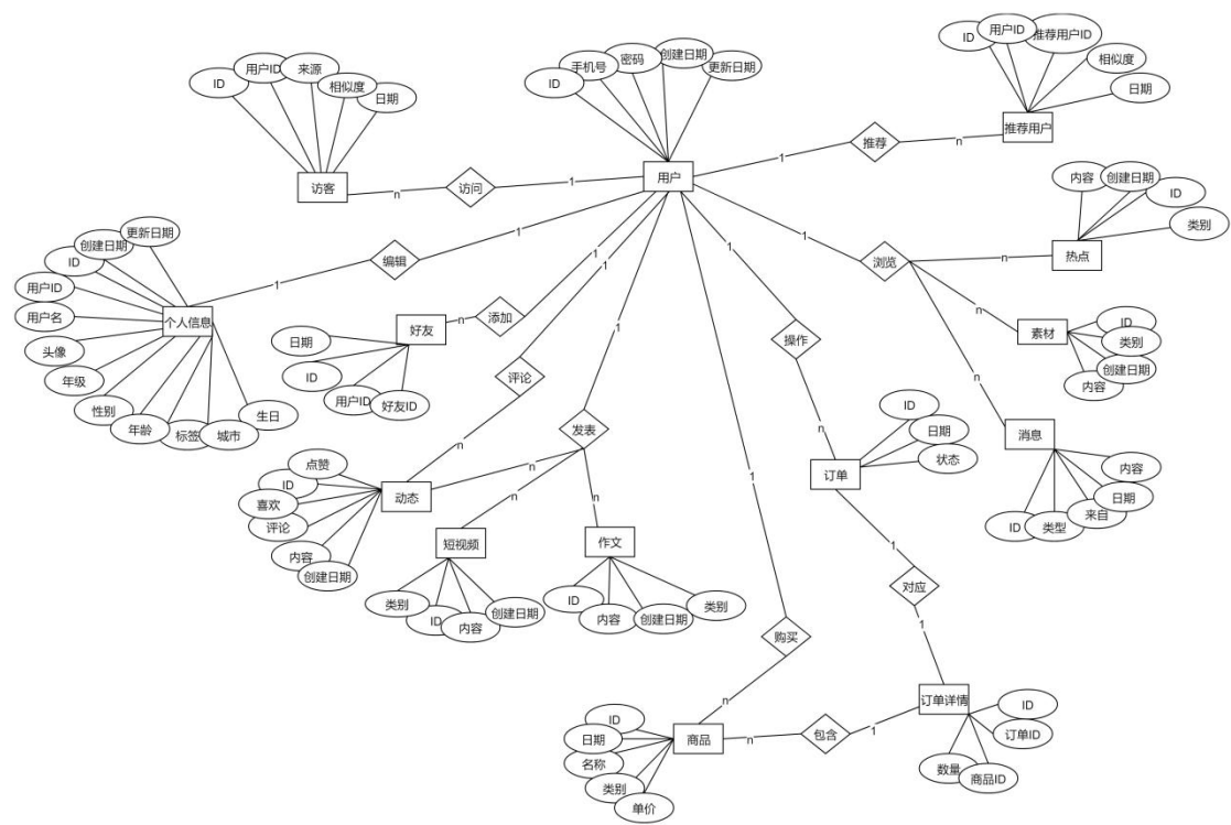
图 B-10 实体关系图
