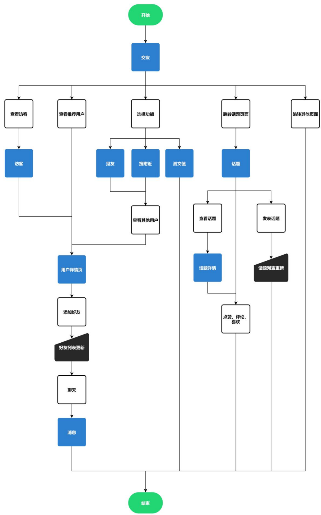
图 B-8 社交功能业务流程图
