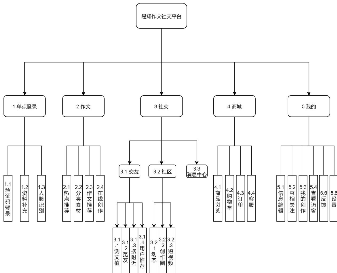
图 2-2 功能模块图
