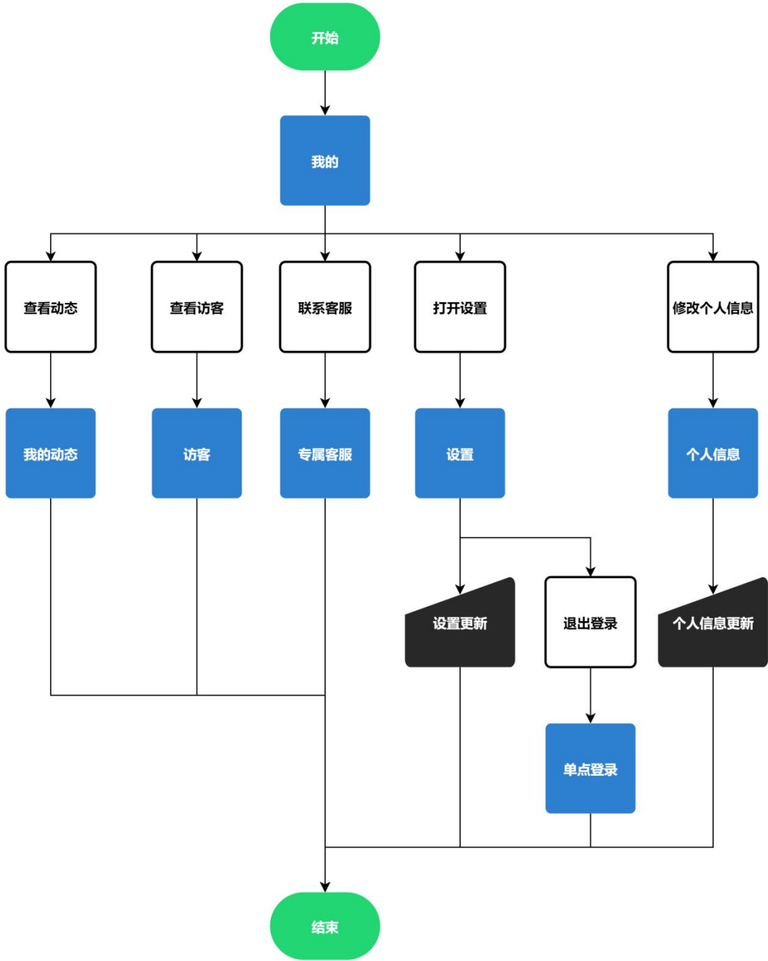
图 B-9 我的页面业务流程图
