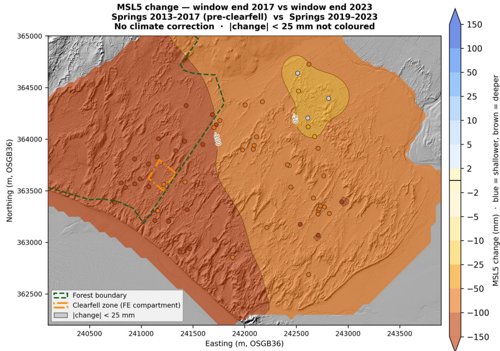
Figur 4. Newid MSL5 2017–2023. n=59 ffynnon; dyfnhaodd 56 >25 mm, 0 yn fwy bas >25 mm. Ffynhonnell: 20_msl5_change_2017_2023.png; Figur 72 yr adroddiad.
