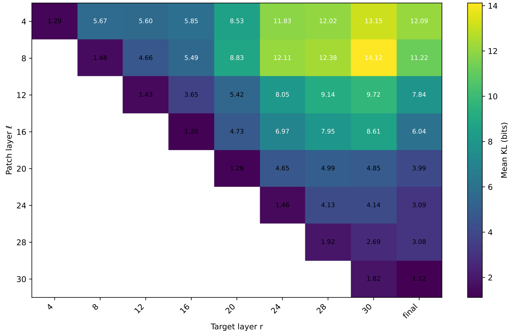
Llama-3.1-8B: SAE reconstruction (Mean KL (bits))
