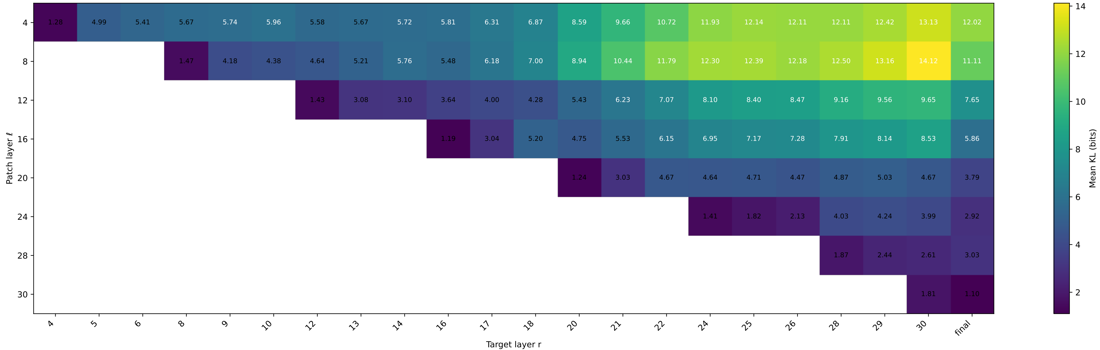
Llama-3.1-8B: SAE reconstruction (Mean KL (bits))
