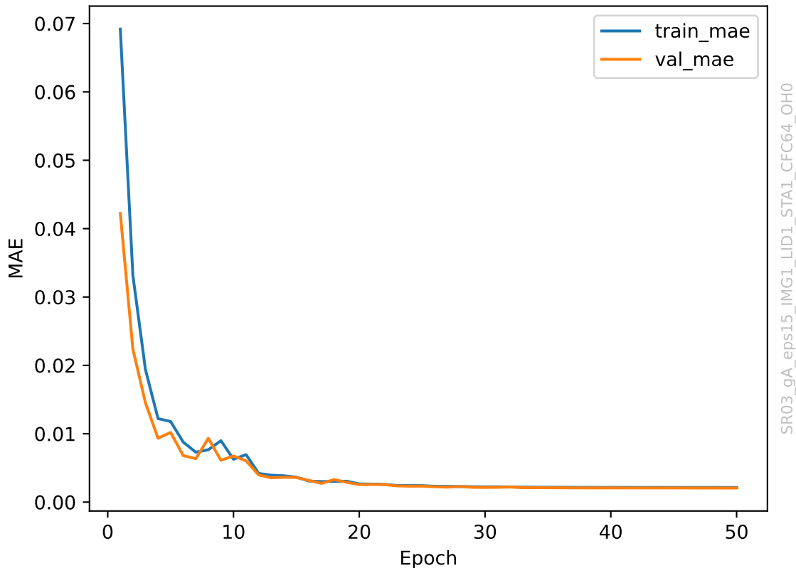
Train vs Val MAE per Epoch
