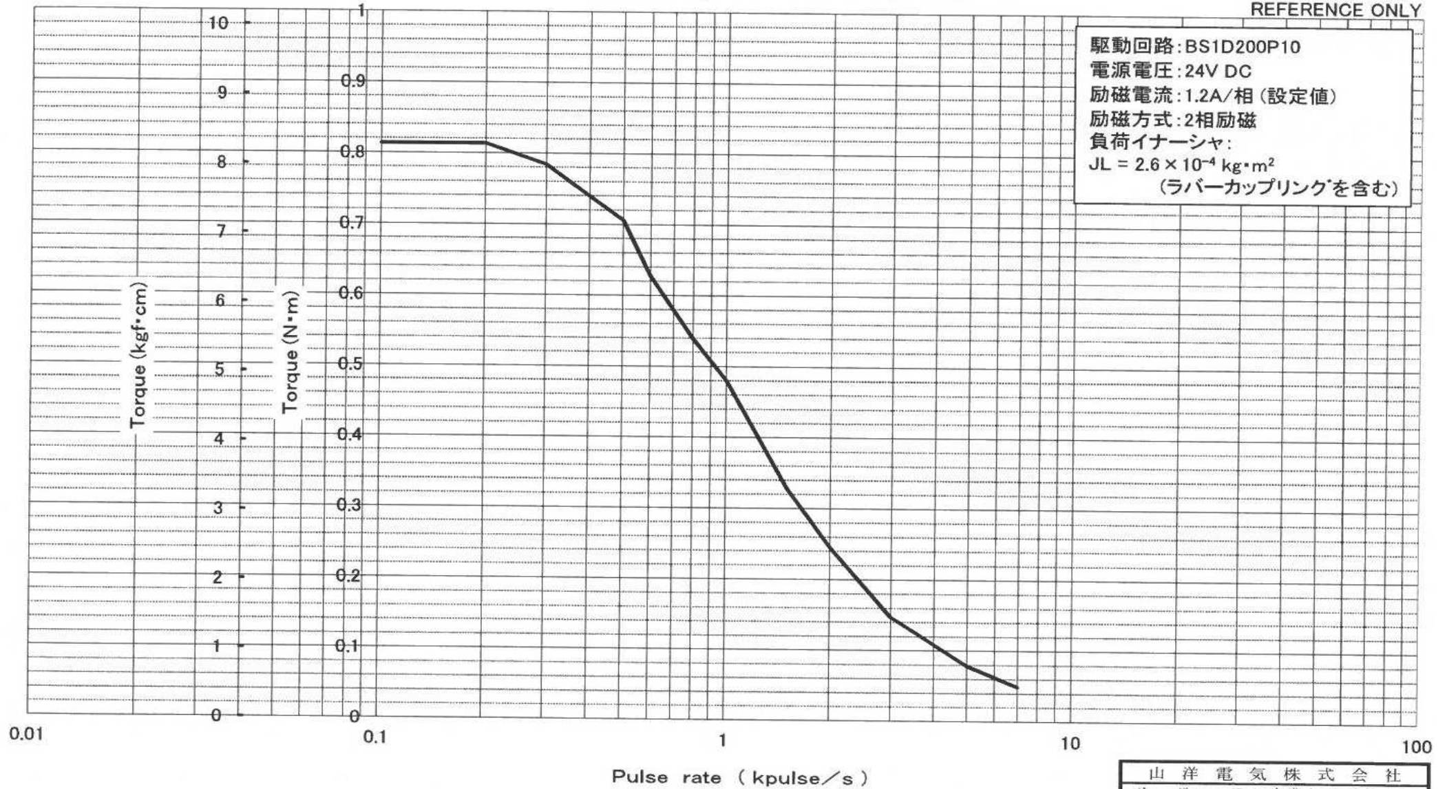
SF2424-12B41 周波数 対 プルアウトトルクカーブ
