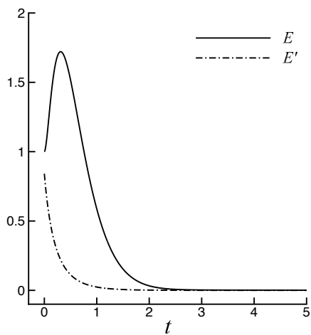
初始能量 E = 1 的能量曲线
