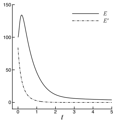
初始能量 E = 100 的能量曲线
