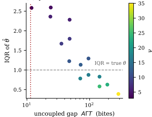
(B) precision
