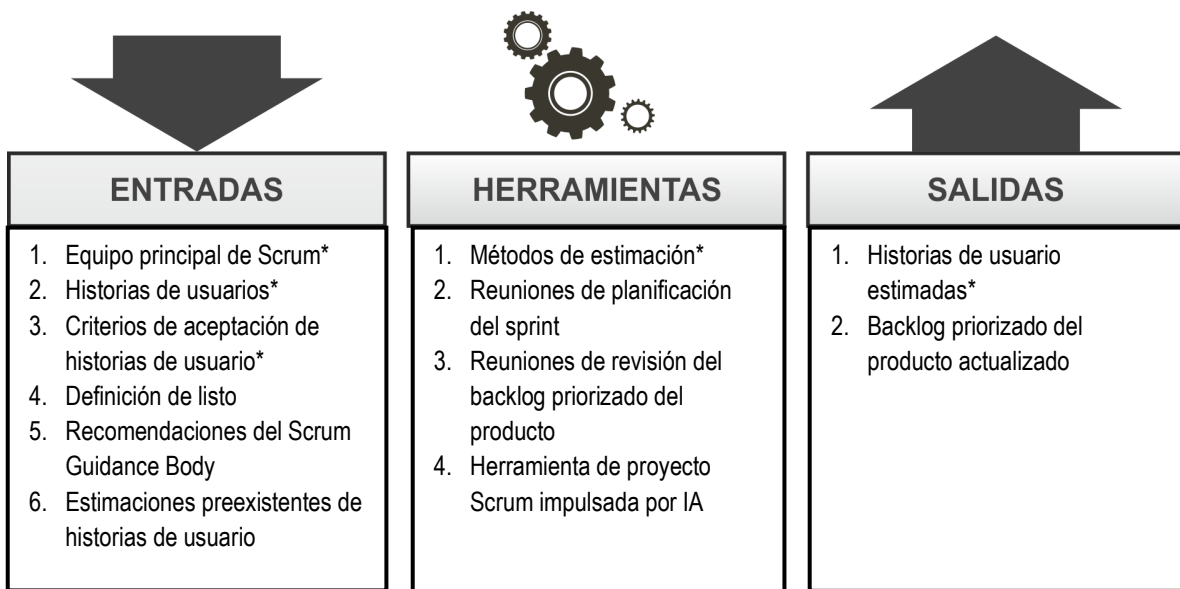
Figura 9-7: Estimar historias de usuario: entradas, herramientas y salidas
