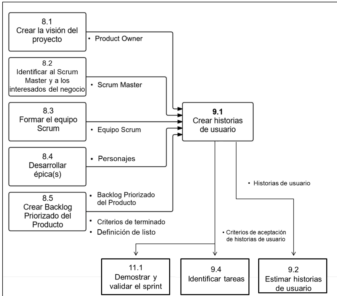
Figura 9-4: Crear historias de usuario: diagrama de flujo
