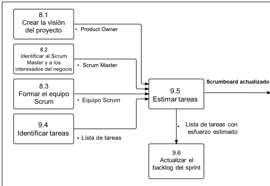
Figura 9-20: Estimar tareas: Diagrama de flujo
