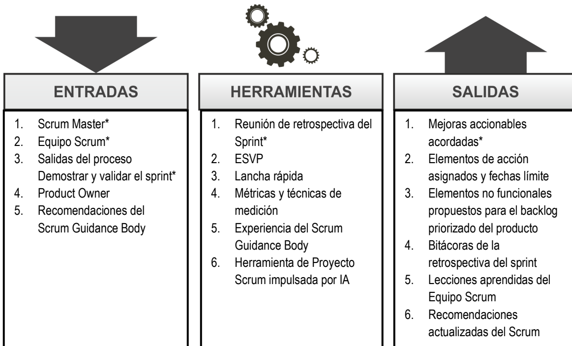
Figura 11-6: Retrospectiva del sprint: entradas, herramientas y salidas
