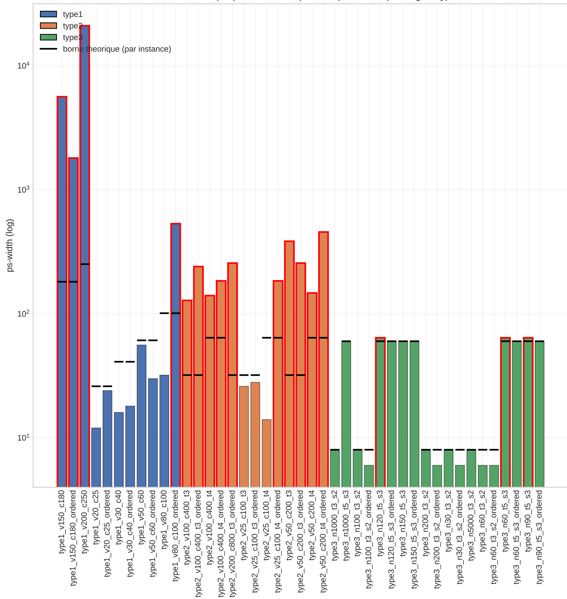
Verification empirique des bornes ps-width par famille (mode greedy)
