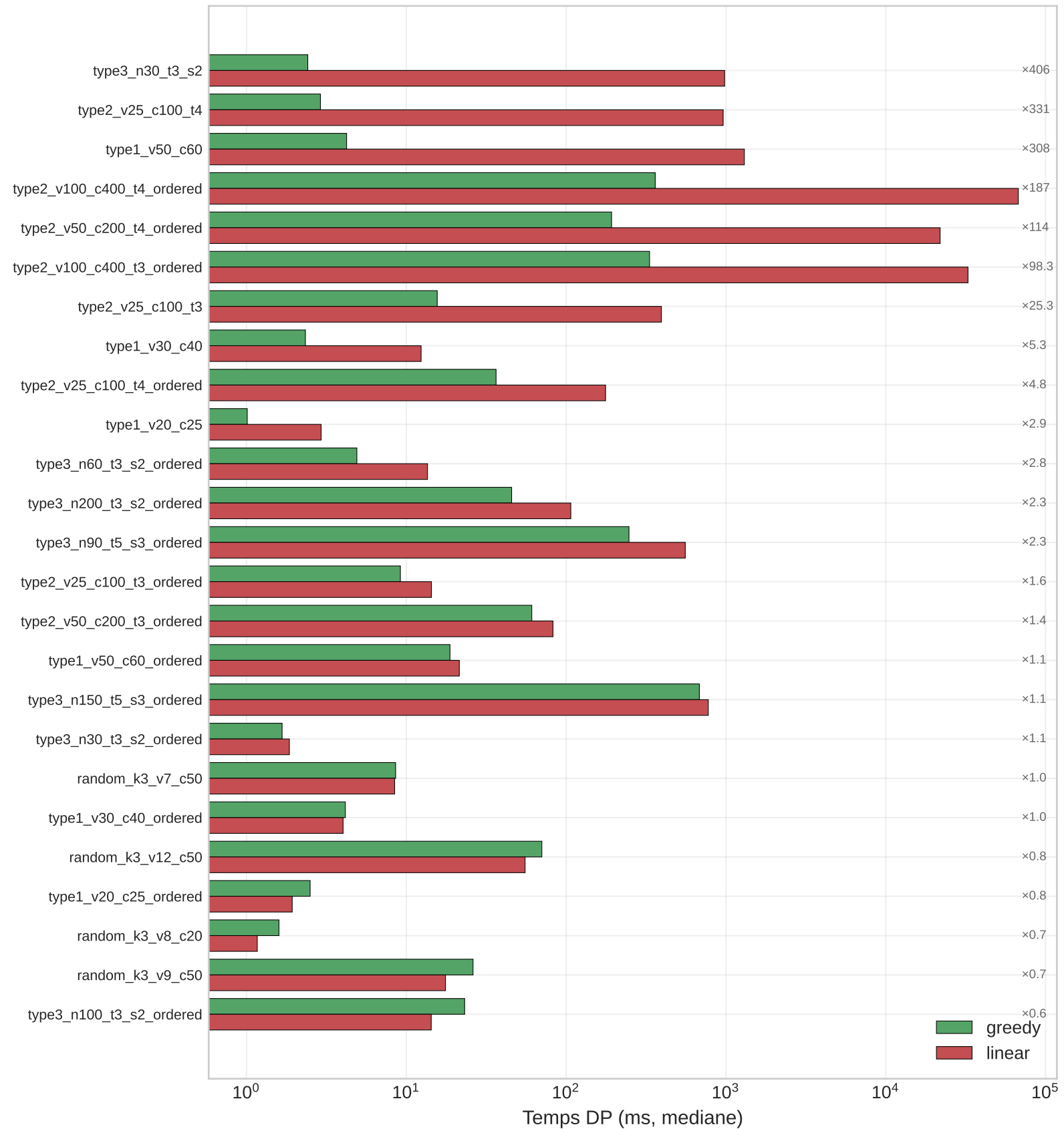
Impact du mode d'arbre sur le temps total DP (mediane sur 3) (top 25 par ratio linear/greedy sur 40 instances)
