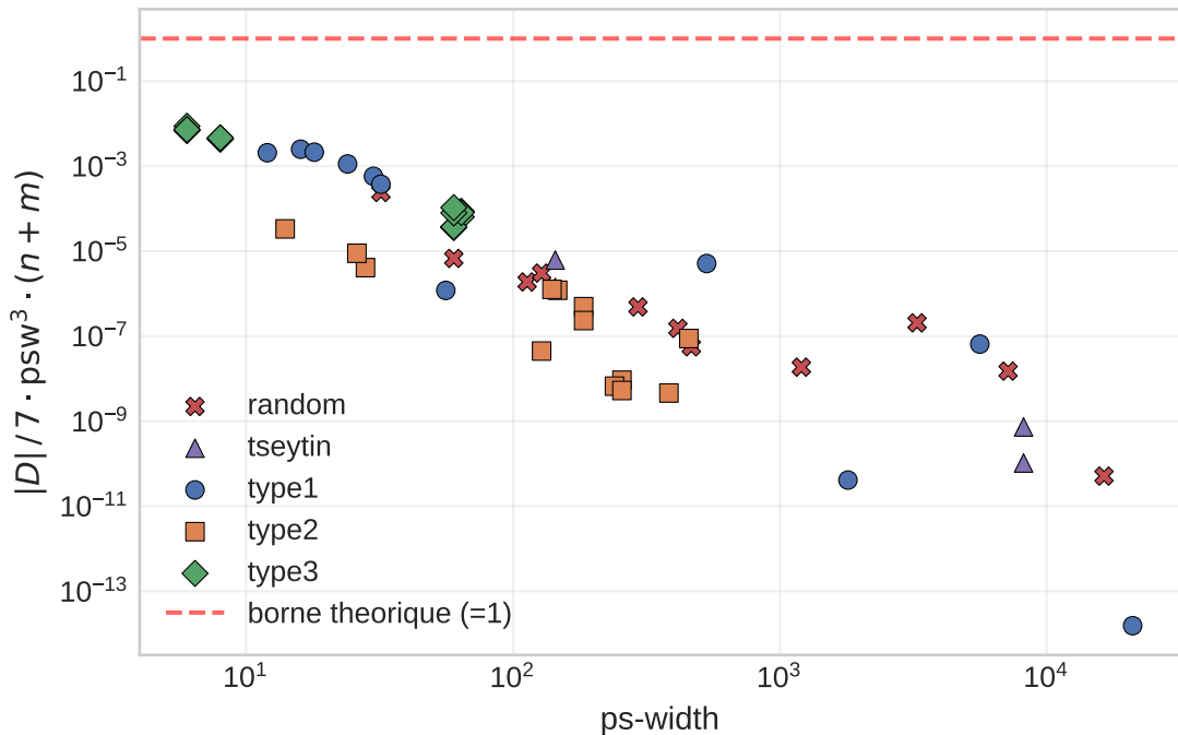
Taille du DAG d-DNNF rapportee a la borne theorique
