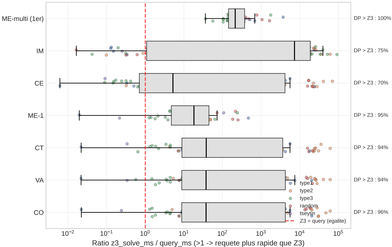
Speedup par requete sur DAG compile vs Z3 froid
