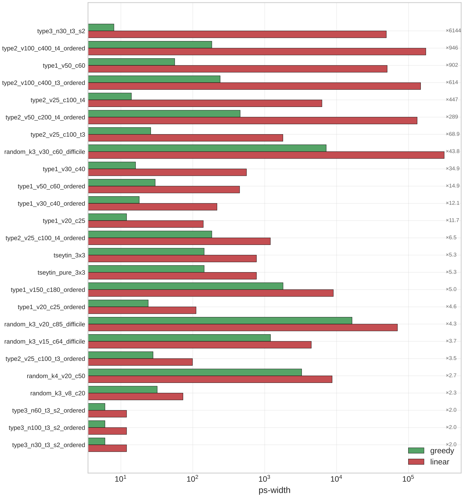
Impact du mode d'arbre sur la ps-width (greedy vs linear) (top 25 par ratio linear/greedy sur 40 instances)
