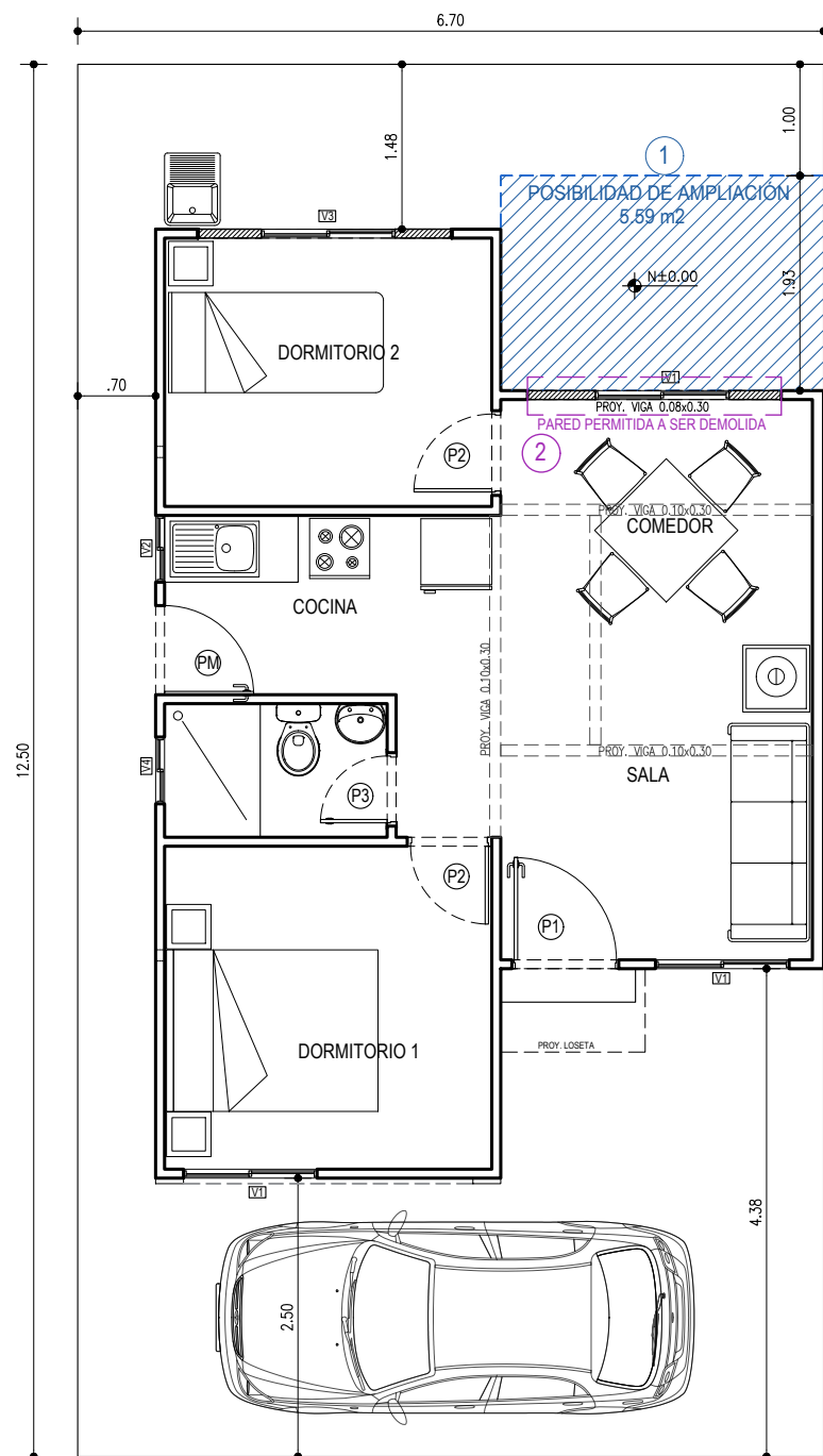
PLANTA BAJA AREA: 41.47 m²
