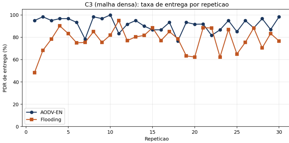
Figura 5.5: Taxa de entrega por repetição no cenário C3 (malha densa): o AODV-EN é mais estável (CV 6,7%) que o flooding (CV 13,2%).
