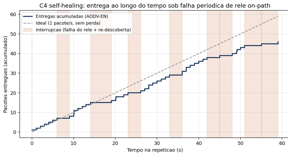
Figura 5.5: Auto-recuperação no cenário C4: pacotes entregues acumulados ao longo de uma repetição. Os patamares (faixas destacadas) coincidem com a queda do relé on-path ; a retomada da entrega evidencia a re-descoberta de rota pelo relé alternativo.
