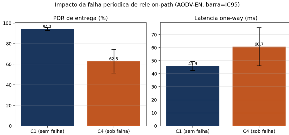
Figura 5.3: Impacto da falha periódica de um relé on-path : PDR de entrega e latência do AODV-EN no cenário C1 (sem falha) contra o C4 (sob falha), com barra de IC95.
