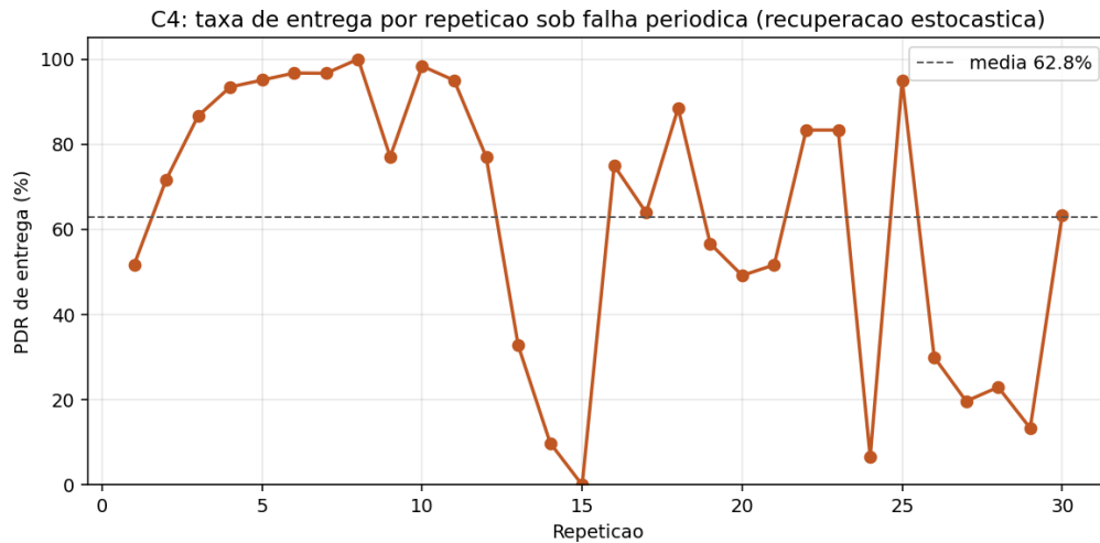
Figura 5.4: Taxa de entrega por repetição no cenário C4: a alta variabilidade reflete a recuperação estocástica diante da falha periódica do relé.
