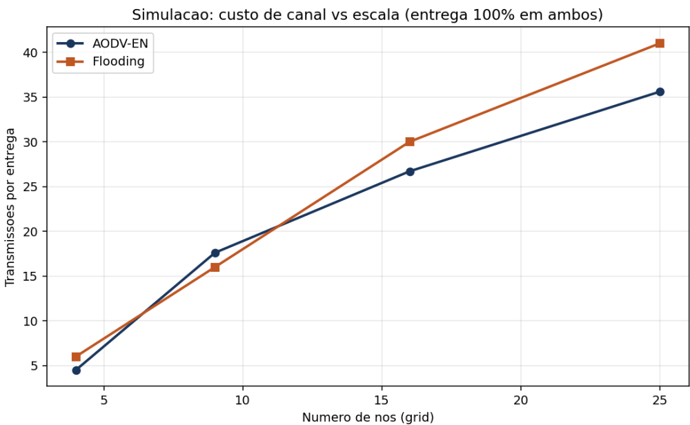
Figura 5.3: Transmissões por pacote entregue em função do número de nós (simulação).
