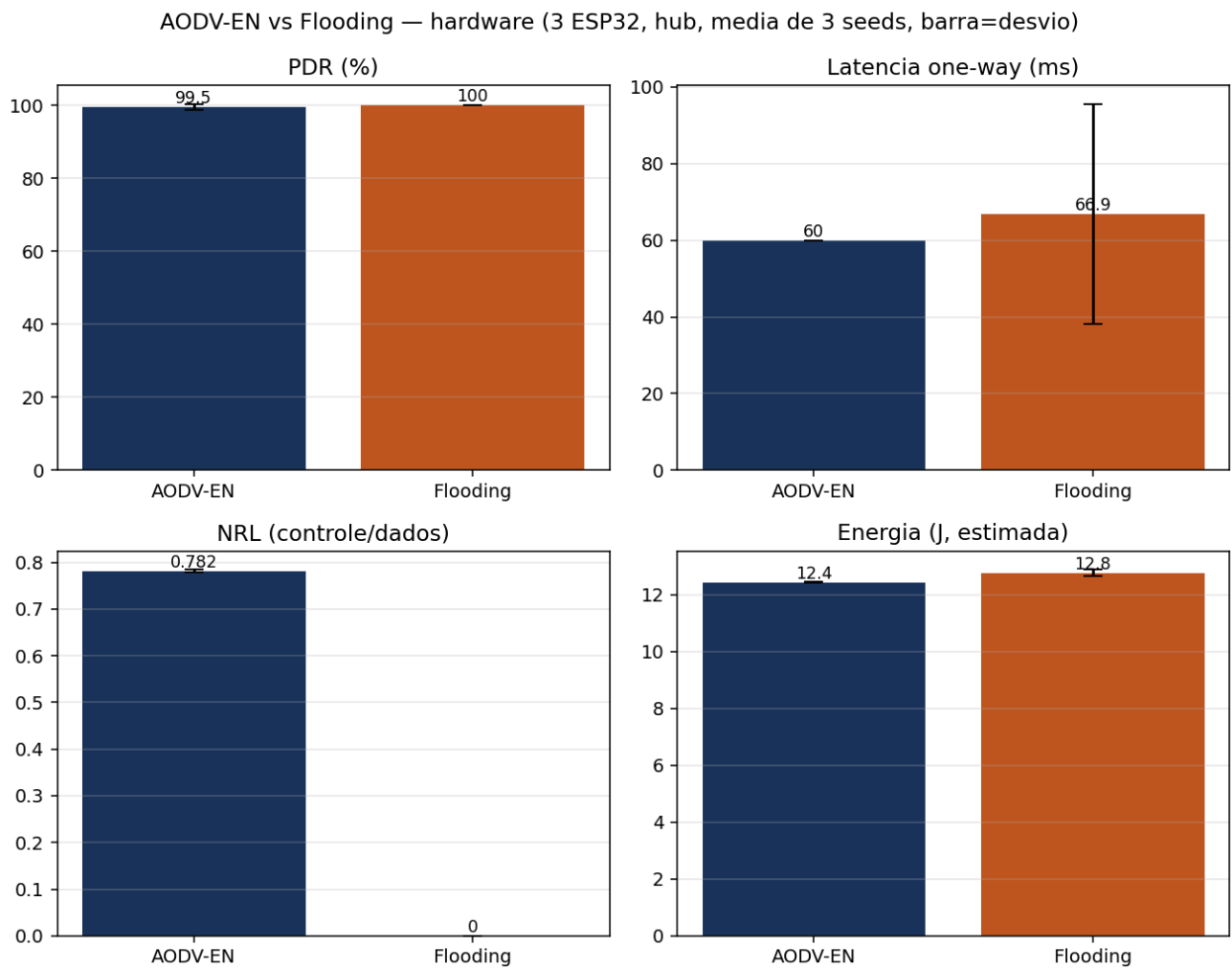
Figura 1 — Quatro métricas do TCC no hardware (3 ESP32, hub), média de 3 seeds; barras de erro = desvio-padrão. PDR ~empate (ambos \approx 100\% ); latência do flooding com grande dispersão (outlier do seed 3); NRL do flooding = 0 (sem controle de roteamento); energia ligeiramente maior no flooding.
