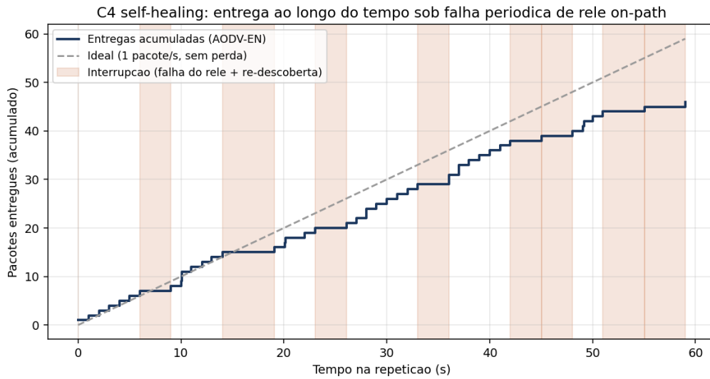
Figura 5.3: Auto-recuperação no cenário C4: pacotes entregues acumulados ao longo de uma repetição. Os patamares (faixas destacadas) coincidem com a queda do relé on-path ; a retomada da entrega evidencia a re-descoberta de rota pelo relé alternativo.
