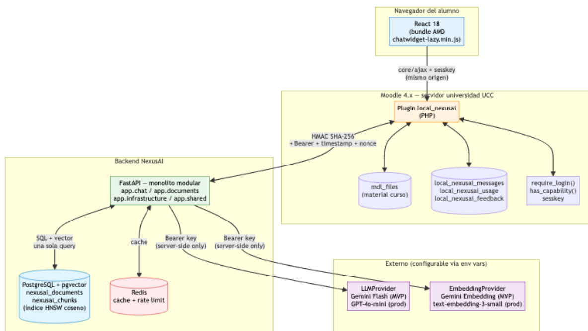
Figura 1. Diagrama de componentes de NexusAI (navegador, plugin Moodle, backend y servicios externos). Fuente: elaboración propia (docs/diagrams/architecture.md). Texto alternativo: esquema de tres capas que conecta el navegador con el plugin PHP, este con el backend FastAPI, y el backend con la base de datos vectorial y los proveedores de LLM y embeddings.
