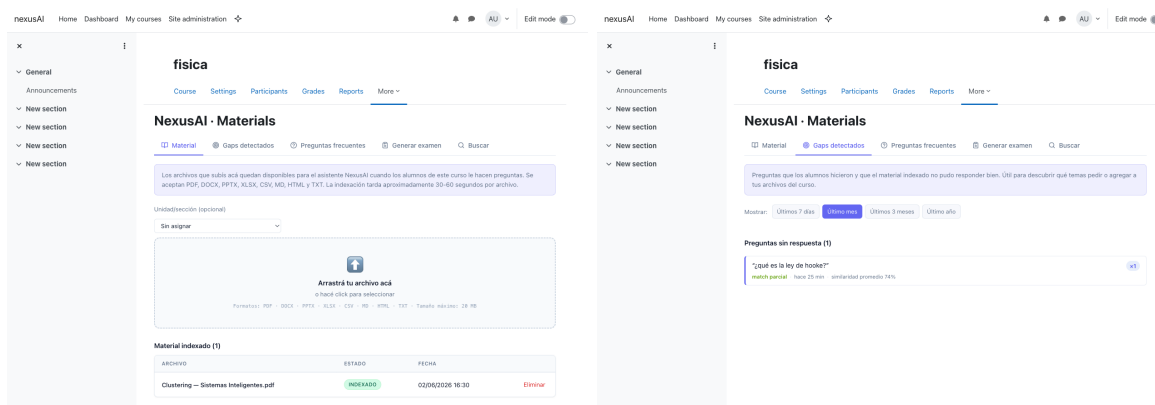
Figura 2c/2d. Panel del docente: gestión de material indexado (izquierda) y repor-
