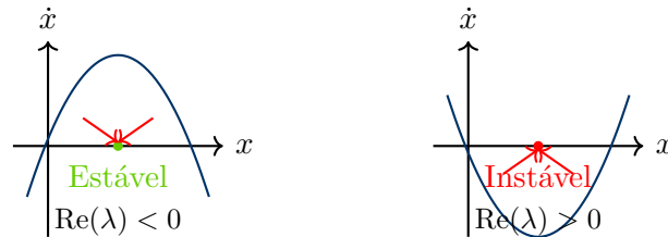
Figura 2.4: Classificação de pontos de equilíbrio unidimensionais pelo sinal de \dot{x} nas vizinhanças. (Esquerda) Equilíbrio estável : \dot{x} > 0 à esquerda e \dot{x} < 0 à direita — perturbações convergem. (Direita) Equilíbrio instável : \dot{x} < 0 à esquerda e \dot{x} > 0 à direita — perturbações divergem. A classificação se estende a sistemas de dimensão n pelos autovalores da jacobiana.
